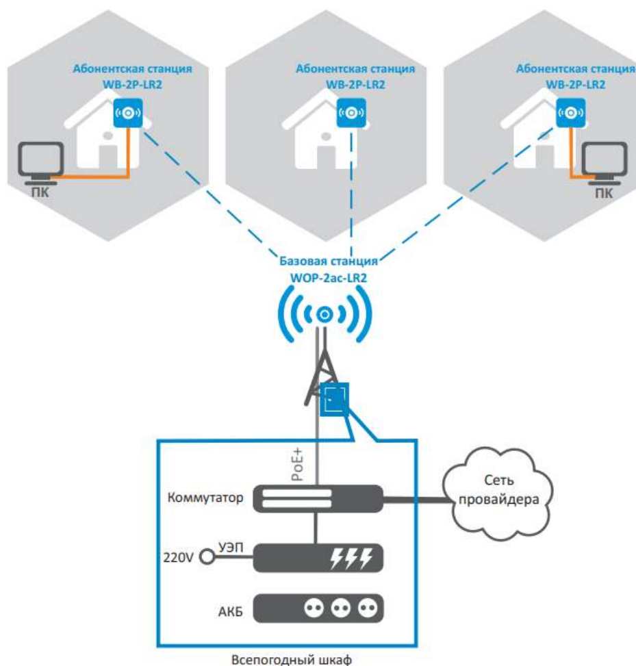
Рисунок 1 – Схема применения WOP-2ac-LR2
