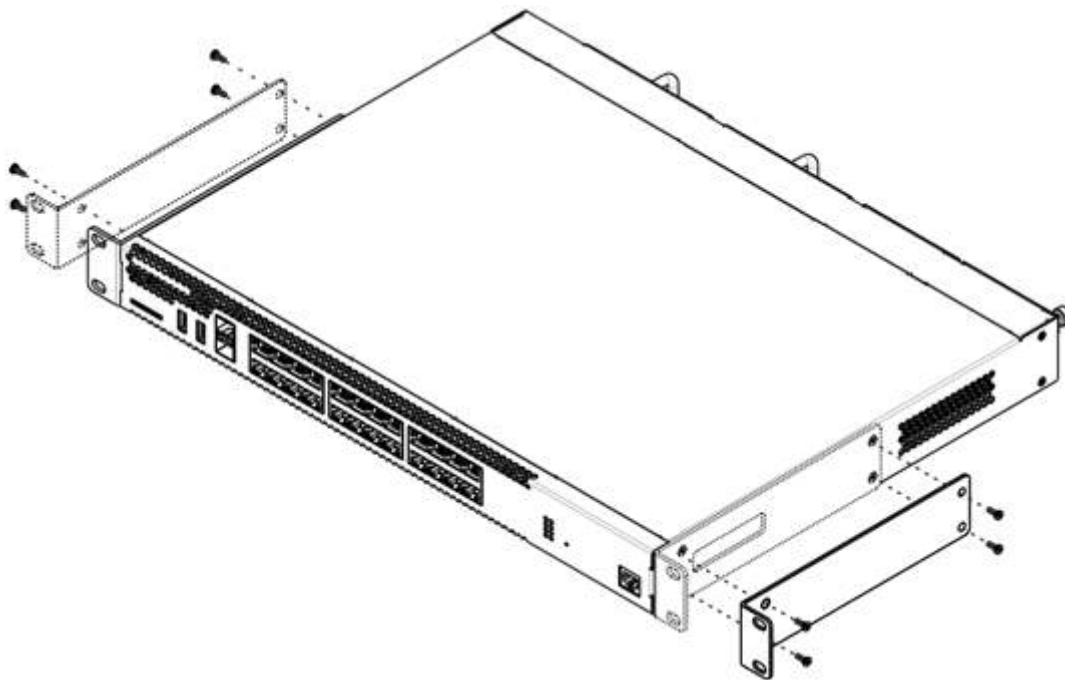
Рисунок 59 – Крепление кронштейнов
