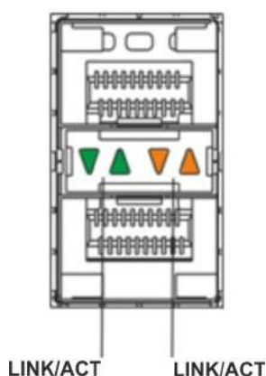
Рисунок 54 – Расположение индикаторов оптических интерфейсов
