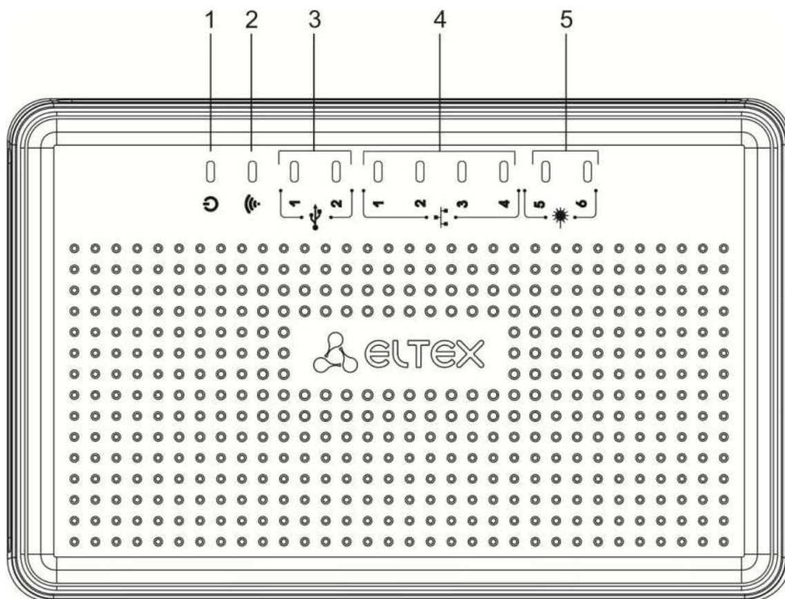
Рисунок 49 – Верхняя панель маршрутизатора ESR-10
