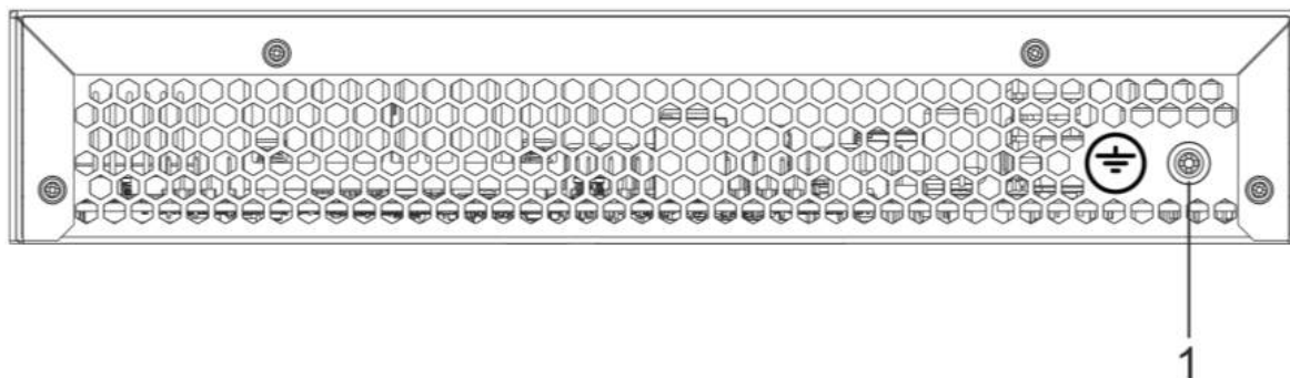
Рисунок 40 – Задняя панель ESR-14VF, ESR-12VF
