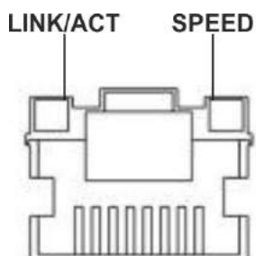
Рисунок 52 – Расположение индикаторов разъема RJ-45
