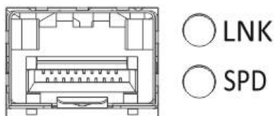
Рисунок 57 – Расположение индикаторов разъема SFP (только для ESR-12VF, ESR-14VF)
