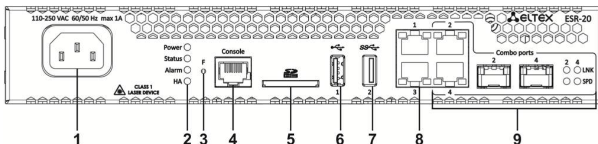
Рисунок 33 – Передняя панель ESR-20
