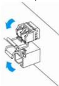
Рисунок 64 – Открытие защелки SFP-трансиверов
