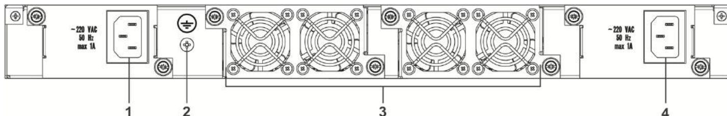
Рисунок 15 – Задняя панель ESR-1511, ESR-1500
