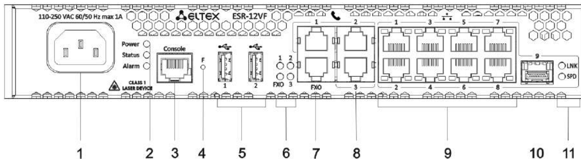
Рисунок 39 – Передняя панель ESR-14VF, ESR-12VF
