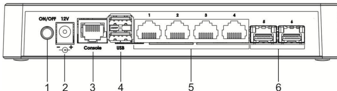
Рисунок 47 – Задняя панель ESR-10
