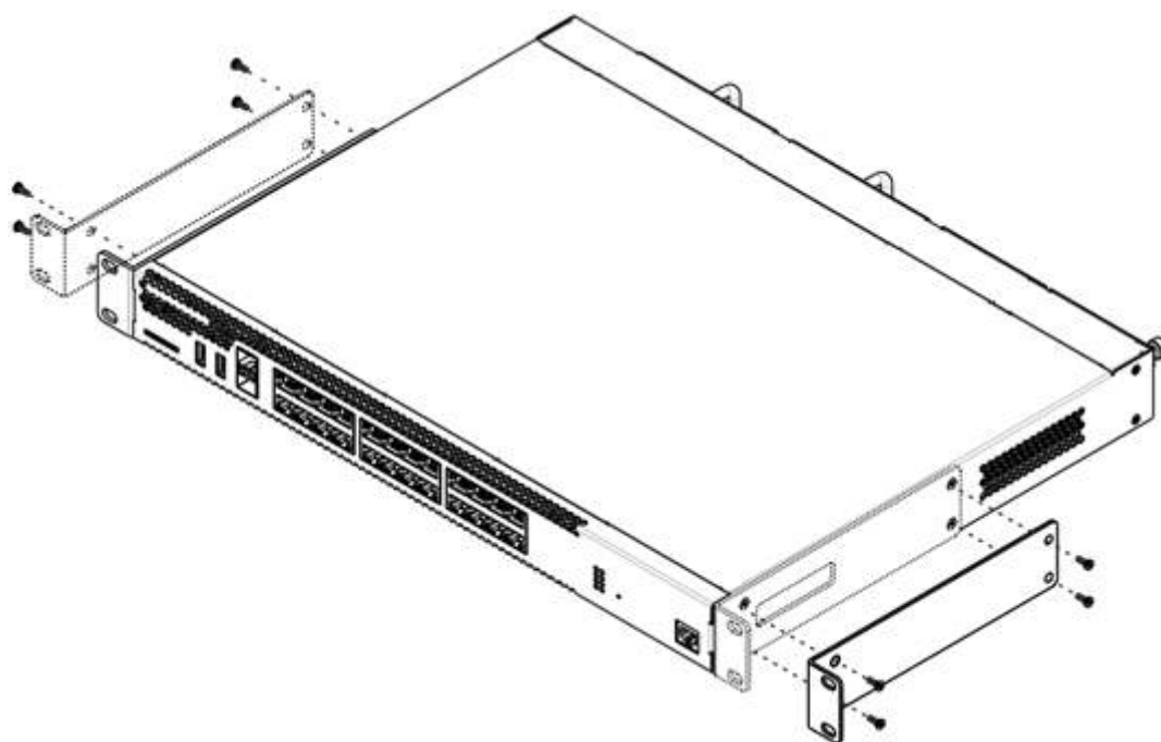
Рисунок 59 – Крепление кронштейнов
