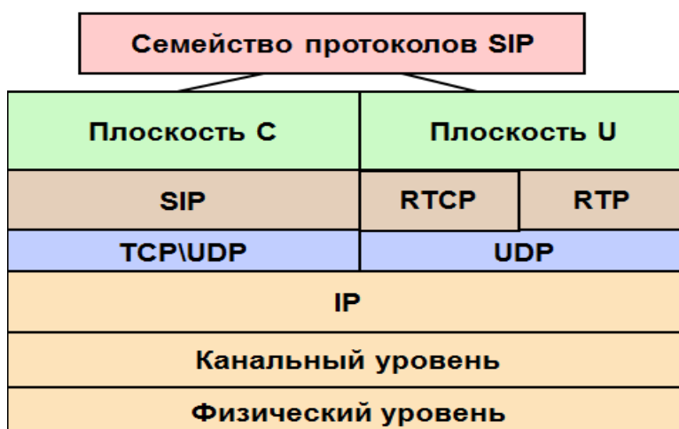
Рисунок 1.23 – Стек протоколов технологии SIP
