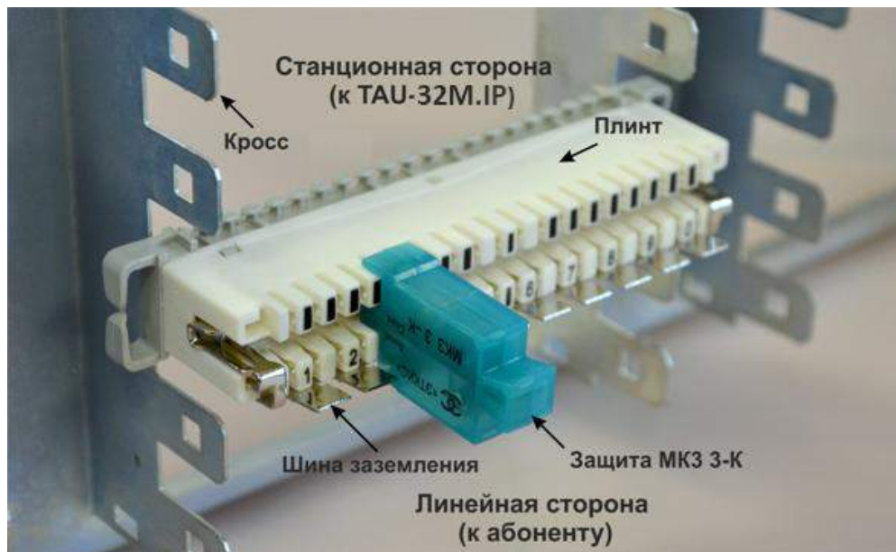
Рисунок 5 – Схема подключения
