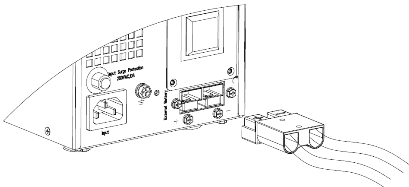
Рис.4 Подключение клемм АКБ
