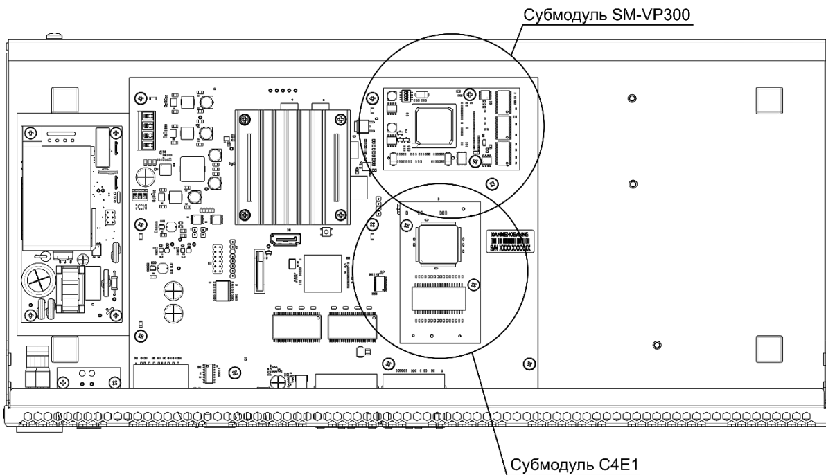
Рисунок 14 – Расположение submodule в SMG-500
