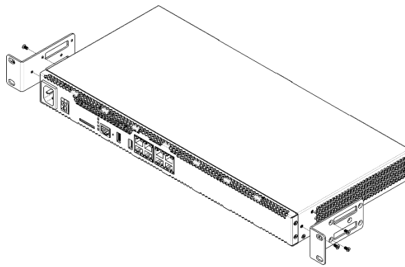
Рисунок 9 – Крепление кронштейнов
