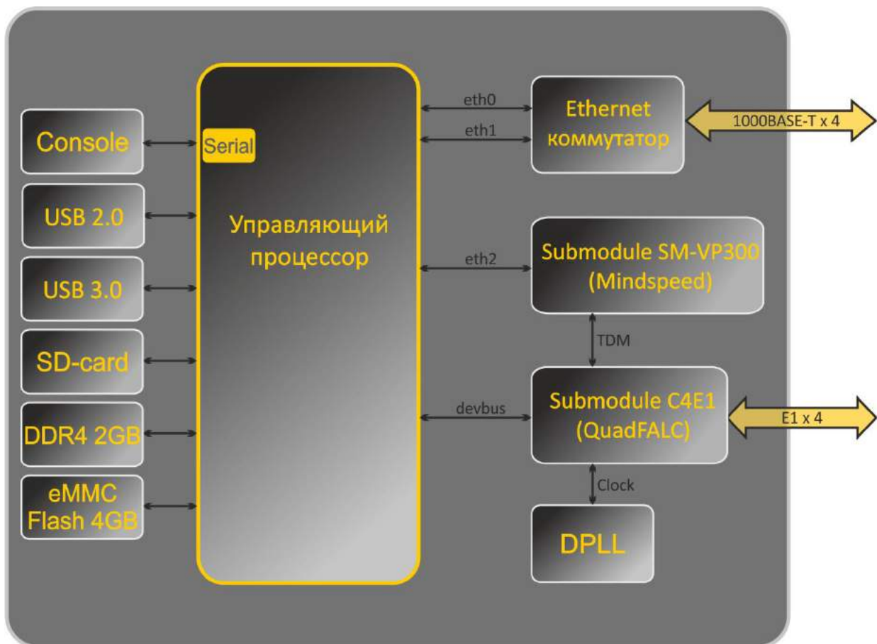
Рисунок 4 – Функциональная схема SMG-500
