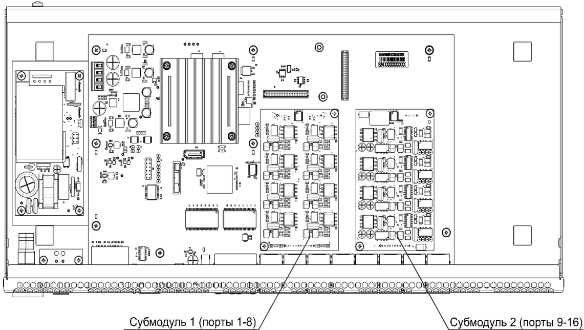
Рисунок 13 – Расположение submodule в SMG-200
