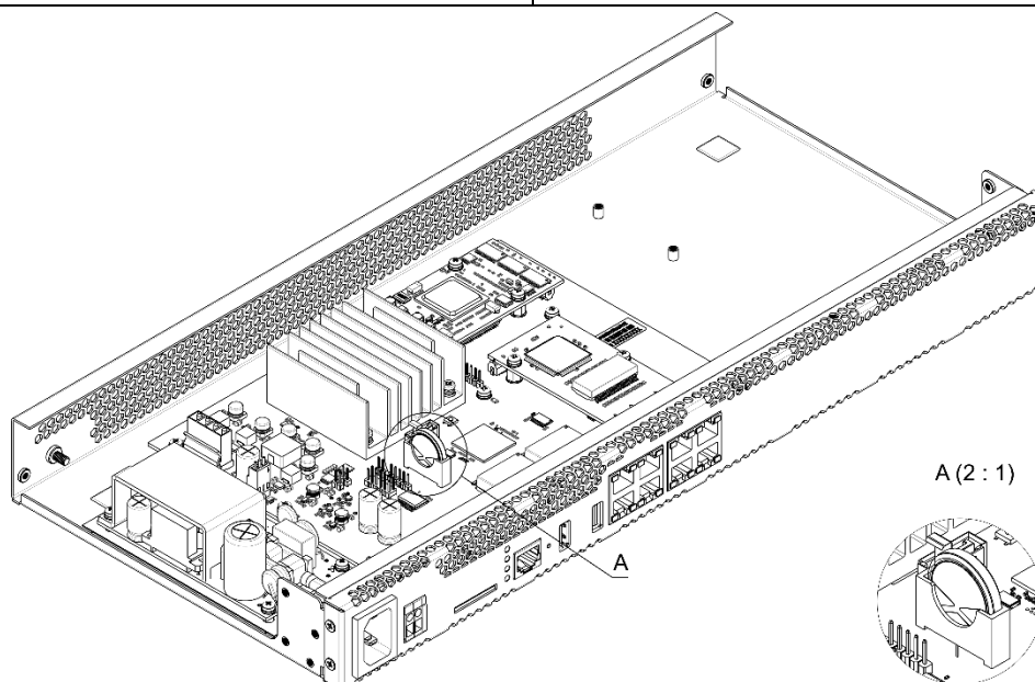
Рисунок 15 – Положение батарейки RTC
