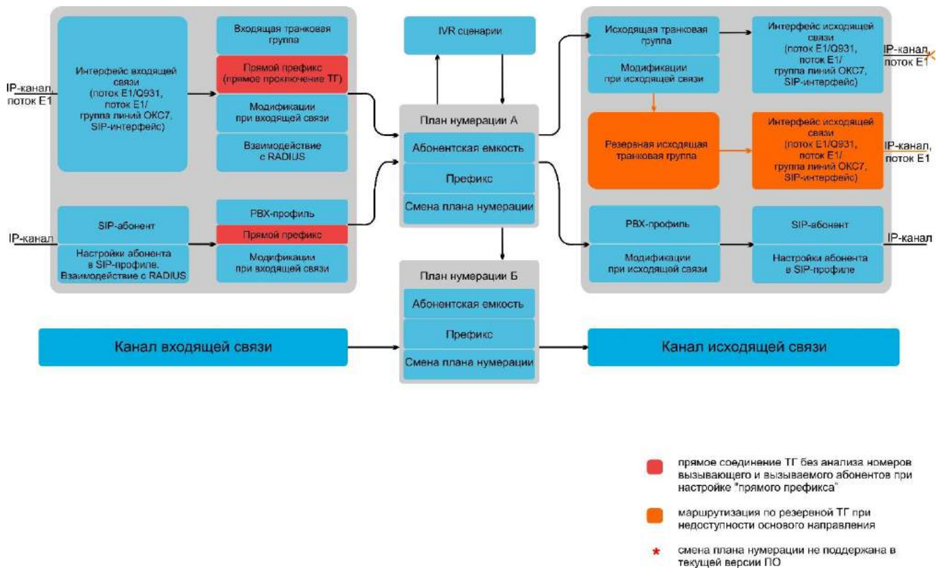
Рисунок 20 – Взаимосвязь параметров маршрутизации, абонентов и СЛ
