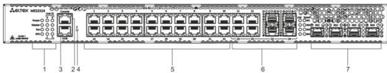
Рисунок 3 — Передняя панель MES3324
