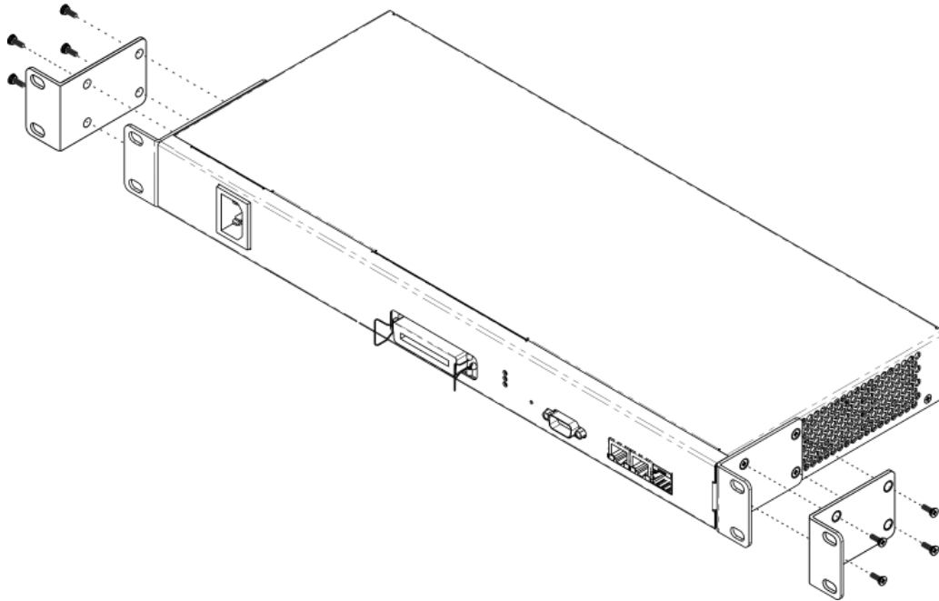
Рисунок 7 – Крепление кронштейнов
