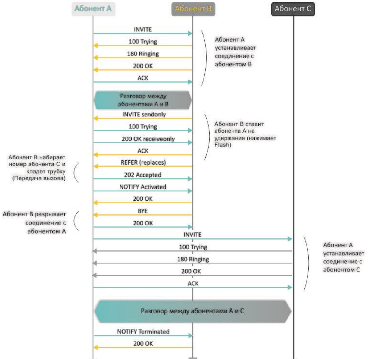
Рисунок 10 – Алгоритм выполнения услуги «Перевод вызова без сопровождения» («Unattended calltransfer») абонентом В по протоколу SIP
