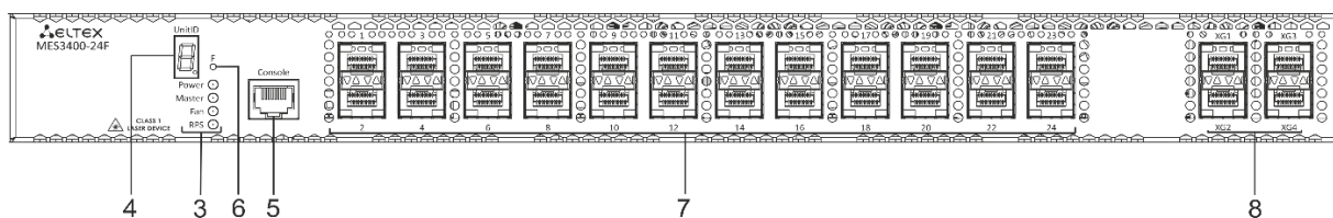
Рисунок 31 – Передняя панель MES3400-24F
