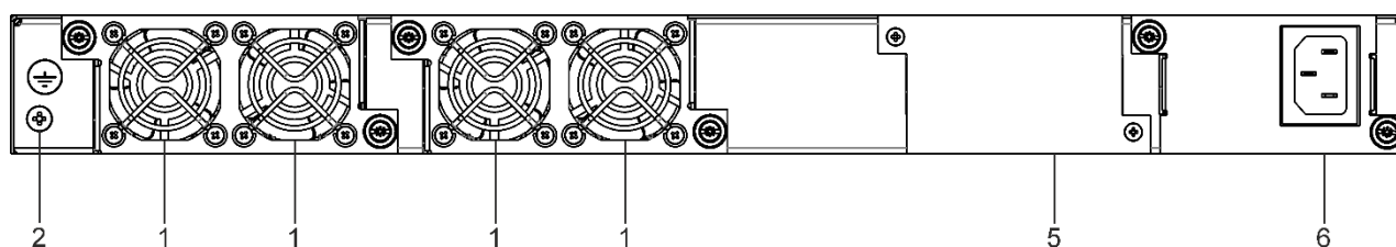
Рисунок 46 — Задняя панель MES3400-24, MES3400I-24, MES3400-48, MES3400-48F
