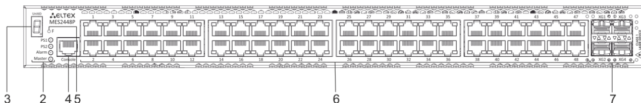
Рисунок 24 – Передняя панель MES2448P
