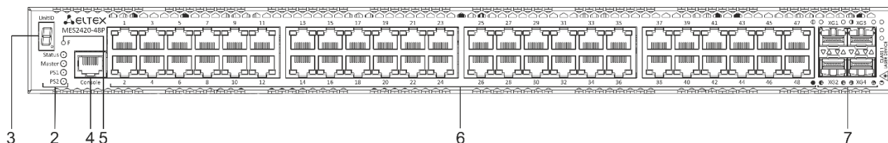
Рисунок 25 – Передняя панель MES2420-48P
