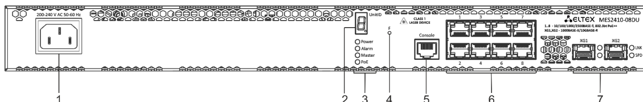
Рисунок 34 – Передняя панель MES2410-08DU
