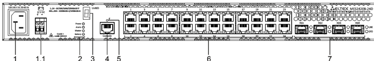
Рисунок 35 – Передняя панель MES2420B-24D
