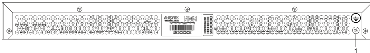
Рисунок 37 – Задняя панель MES1428, MES2428, MES2428T, MES2428B, MES2408IP DC1, MES2408P, MES2424 и MES2424B
