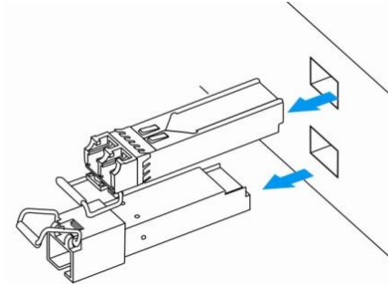
Рисунок 63 – Извлечение SFP-трансиверов
