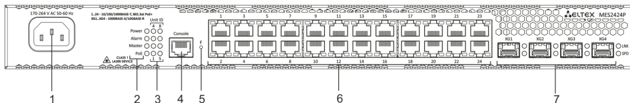
Рисунок 21 – Передняя панель MES2424P
