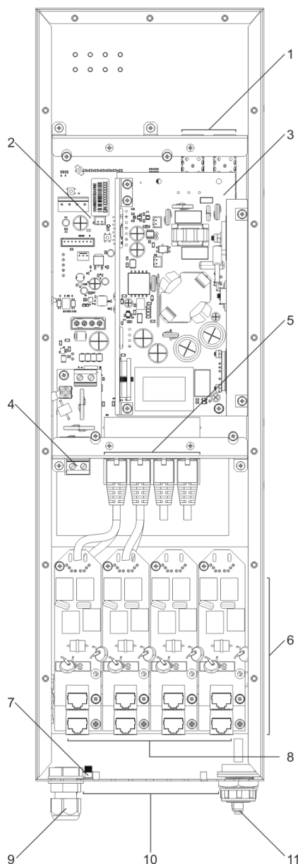
Рисунок 52 – Основные компоненты и разъемы MES3708P
