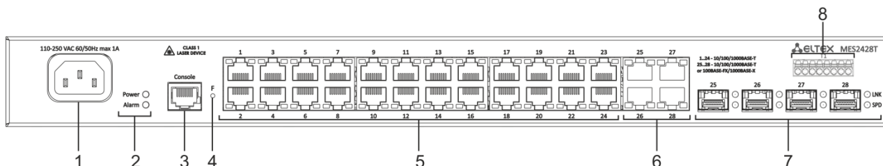
Рисунок 17 – Передняя панель MES2428T
