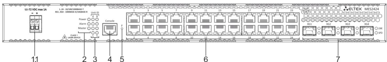
Рисунок 19 – Передняя панель MES2424 DC
