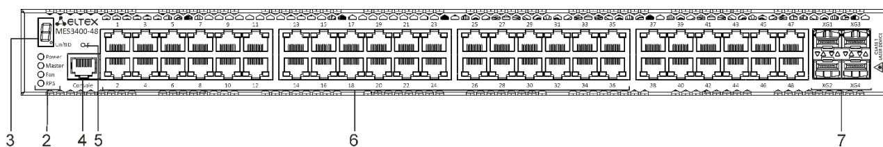
Рисунок 29 – Передняя панель MES3400-48
