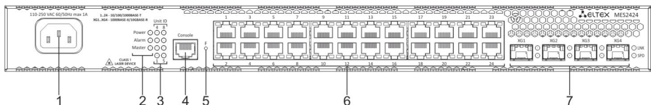
Рисунок 18 – Передняя панель MES2424 AC
