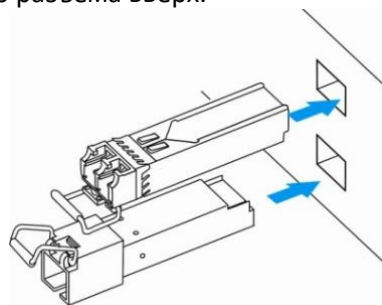
Рисунок 60 – Установка SFP-трансиверов
