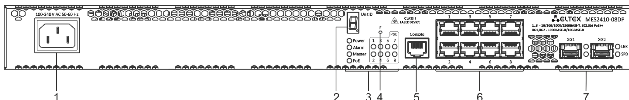
Рисунок 33 – Передняя панель MES2410-08DP
