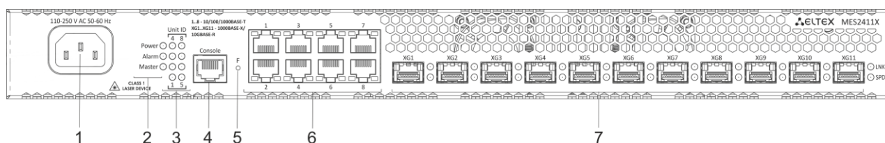
Рисунок 26 – Передняя панель MES2411X
