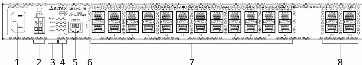
Рисунок 30 – Передняя панель MES2424FB
