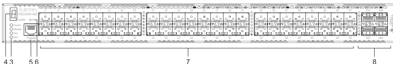
Рисунок 32 – Передняя панель MES3400-48F
