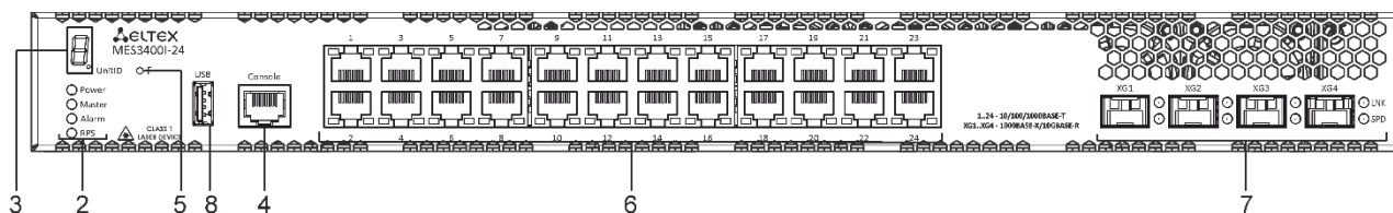
Рисунок 28 – Передняя панель MES3400I-24
