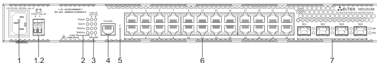
Рисунок 20 – Передняя панель MES2424B
