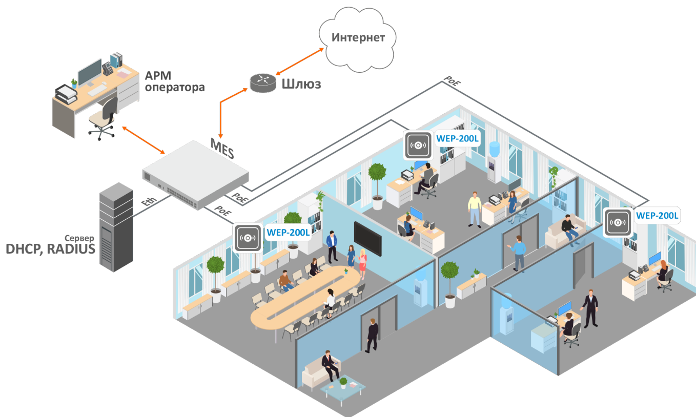
Рисунок 1 — Функциональная схема использования WEP-200L
