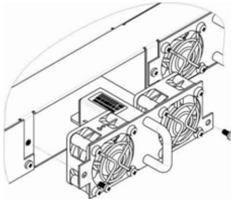
Рисунок 33 – Блок вентиляции SMG-2016. Крепление в корпус
