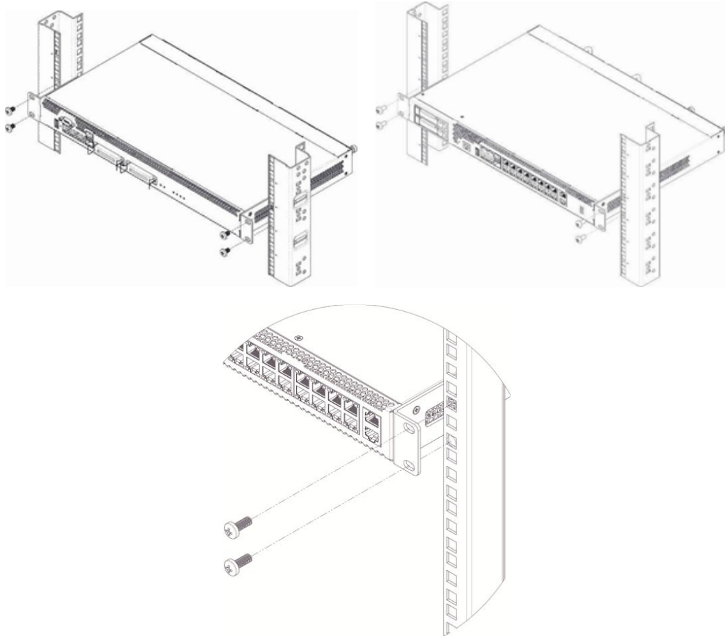
Рисунок 20 – Установка устройства в стойку SMG-1016M (слева), SMG-2016 (справа) и SMG-3016 (внизу)
