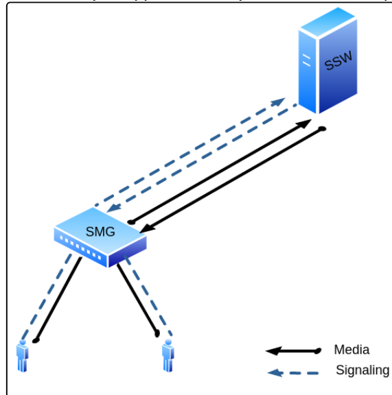
Рисунок 60 – MSR расположен на SSW
