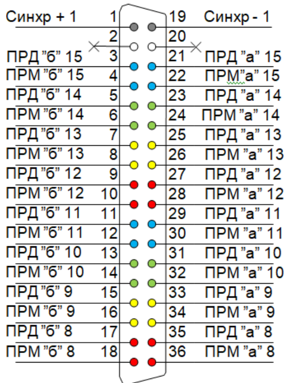
Рисунок 50 – Назначение контактов разъемов E1 Line
