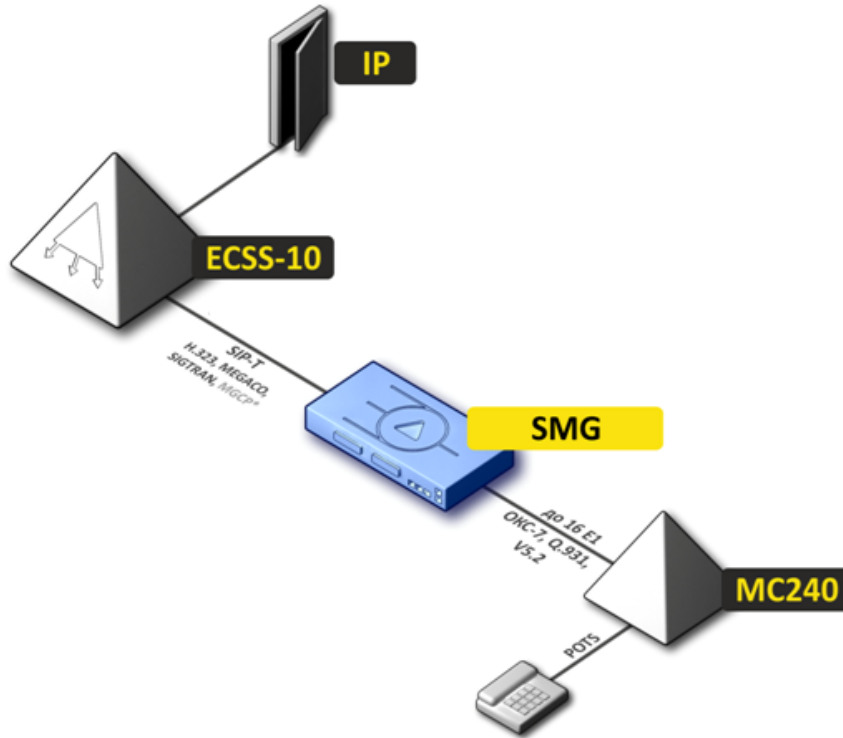
Рисунок 2 – Сопряжение сигнализаций и медиапотоків TDM- и VoIP-сетей
