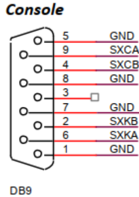
Рисунок 51 – Назначение контактов разъема Console
