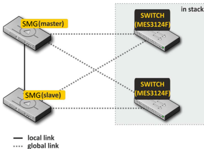
Рисунок 55 – Схема резервирования двумя коммутаторами в стеке
