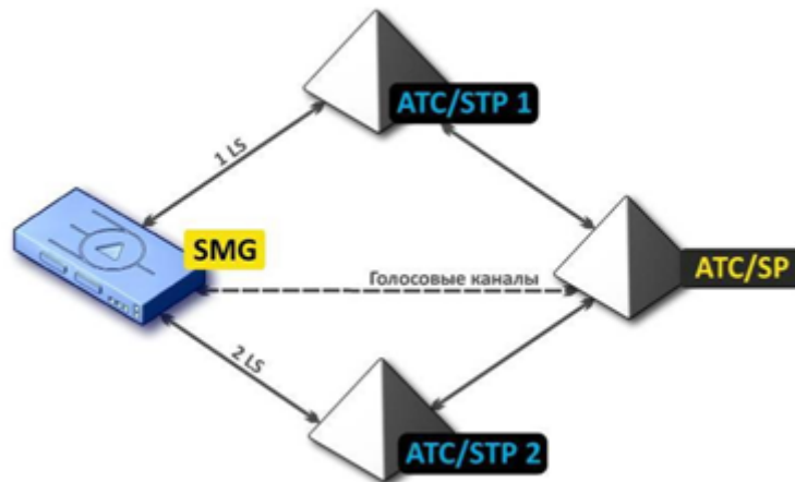
Рисунок 48 – Схема подключения SMG в комбинированном режиме
