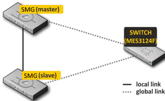
Рисунок 54 – Схема резервирования с одним коммутатором
