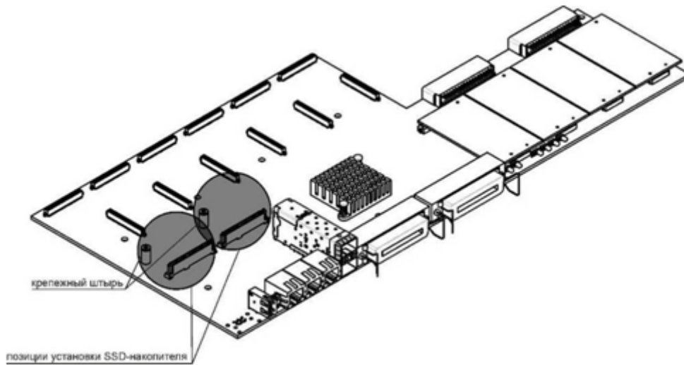
Рисунок 37 – Установка SSD-накопителя
