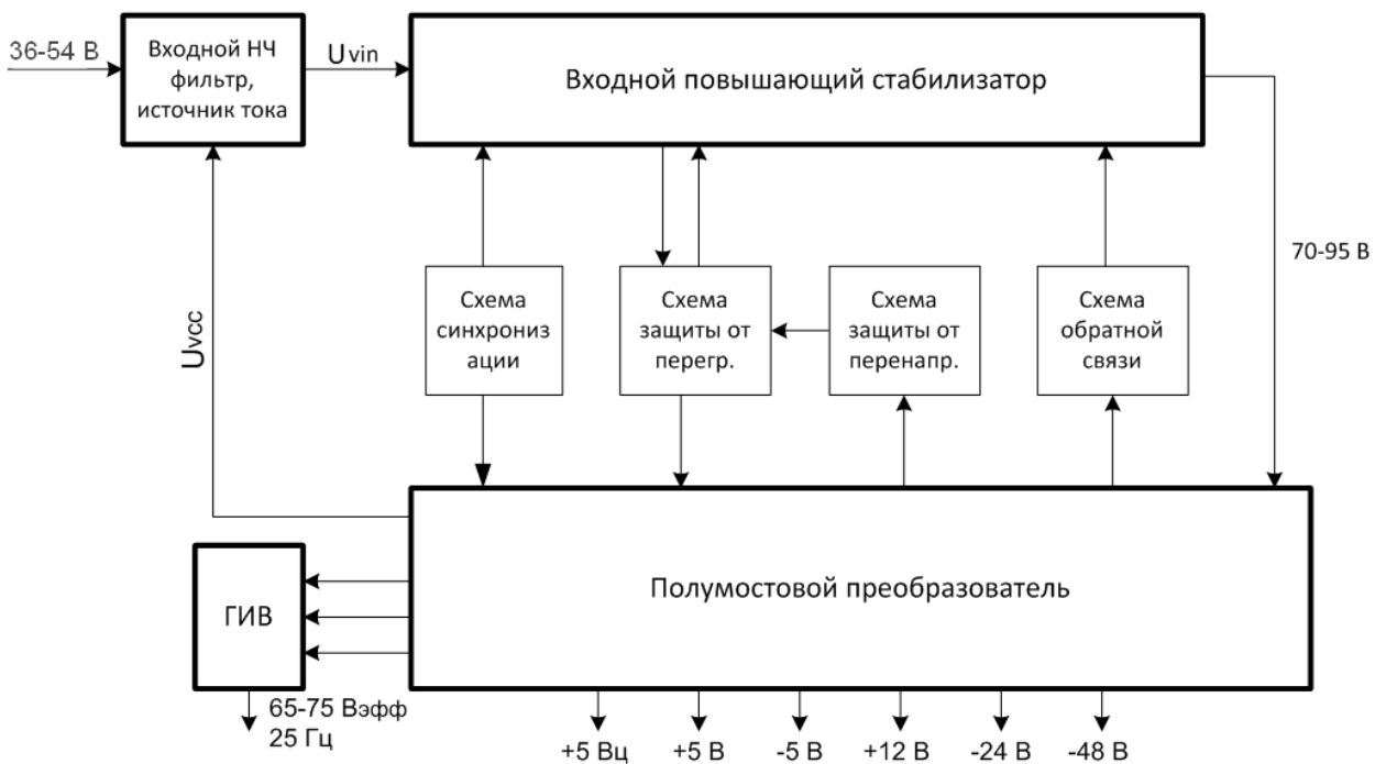
Рисунок 18 – Блок питания
