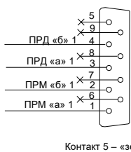
Модуль СОРМ
