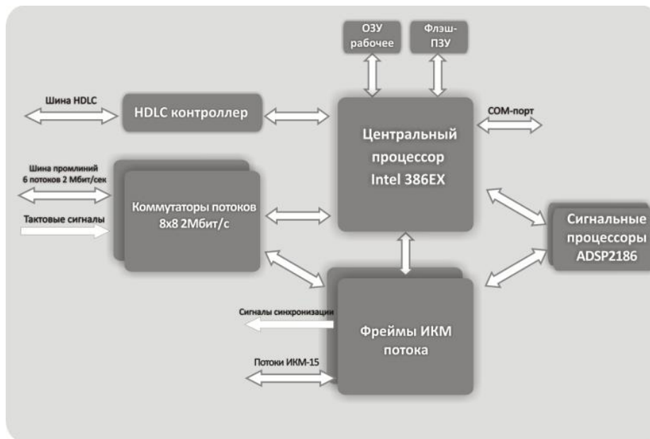
Рисунок 12 – Функциональная схема модуля 2И15
