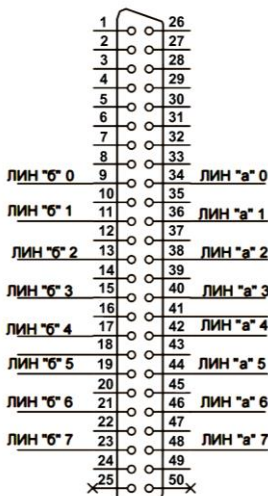
Модуль 8МБ
