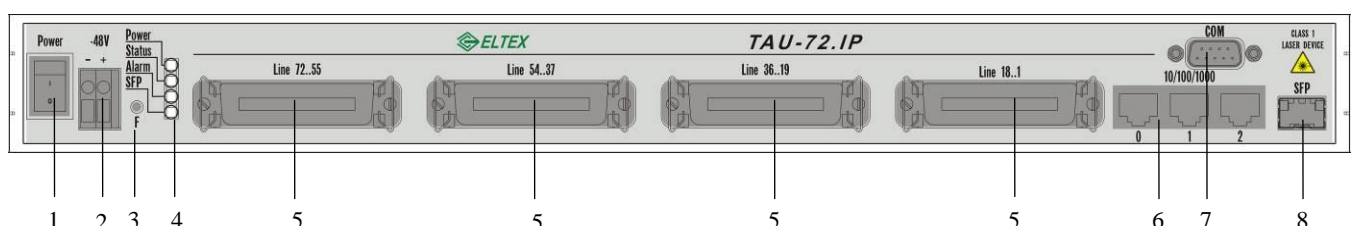
Рисунок 3а – Внешний вид передней панели TAU-72.IP v2.0
