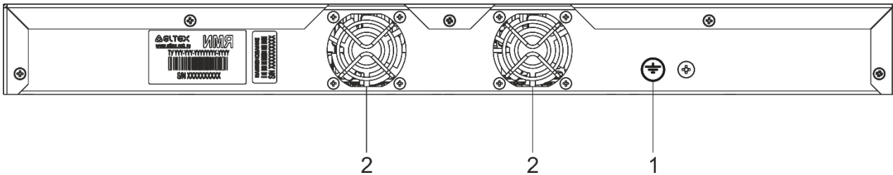
Рисунок 31 — Задняя панель MES2324P
