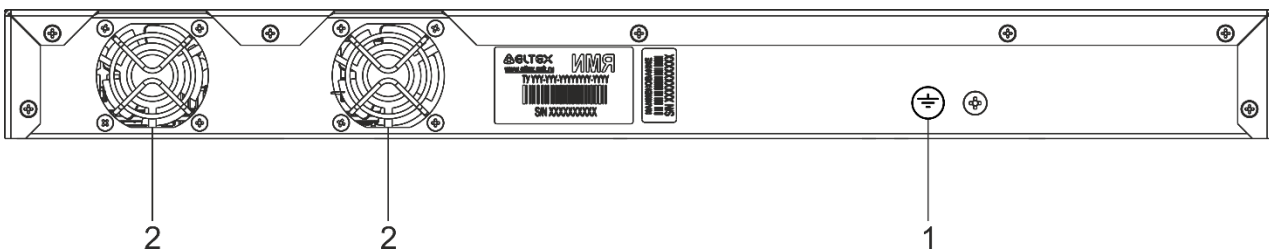
Рисунок 32 — Задняя панель MES2324P ACW
