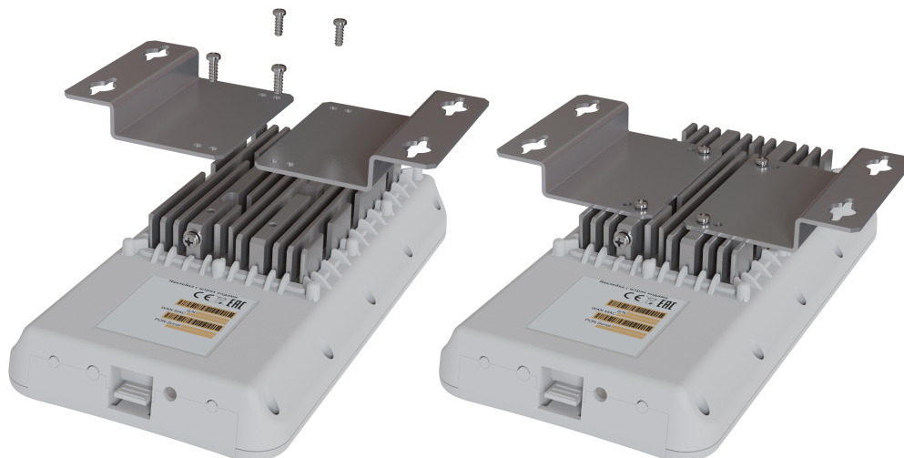
Рисунок 12— Крепление кронштейна к устройству
