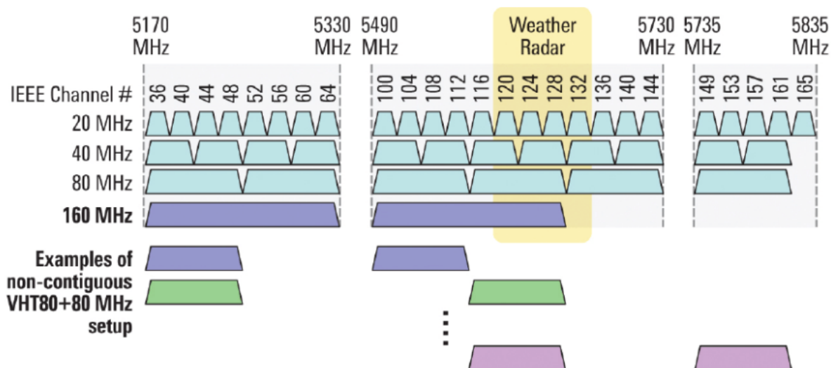
Рисунок 9 — Каналы, используемые в диапазоне 5 ГГц при ширине канала 20, 40, 80 МГц
