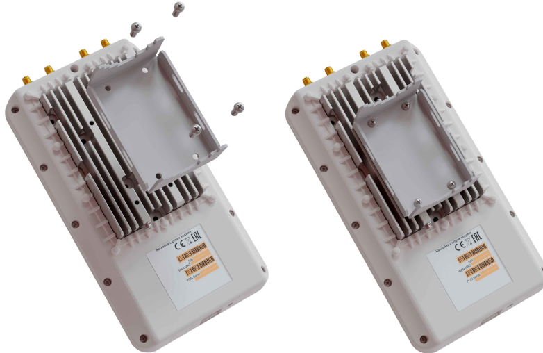
Рисунок 10 — Крепление кронштейна к устройству
