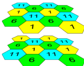
Рисунок 8 — Схема распределения каналов между соседними точками доступа, расположенными между этажами
