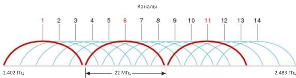
Рисунок 6 – Общая диаграмма перекрытия частотных каналов в 2.4 ГГц
