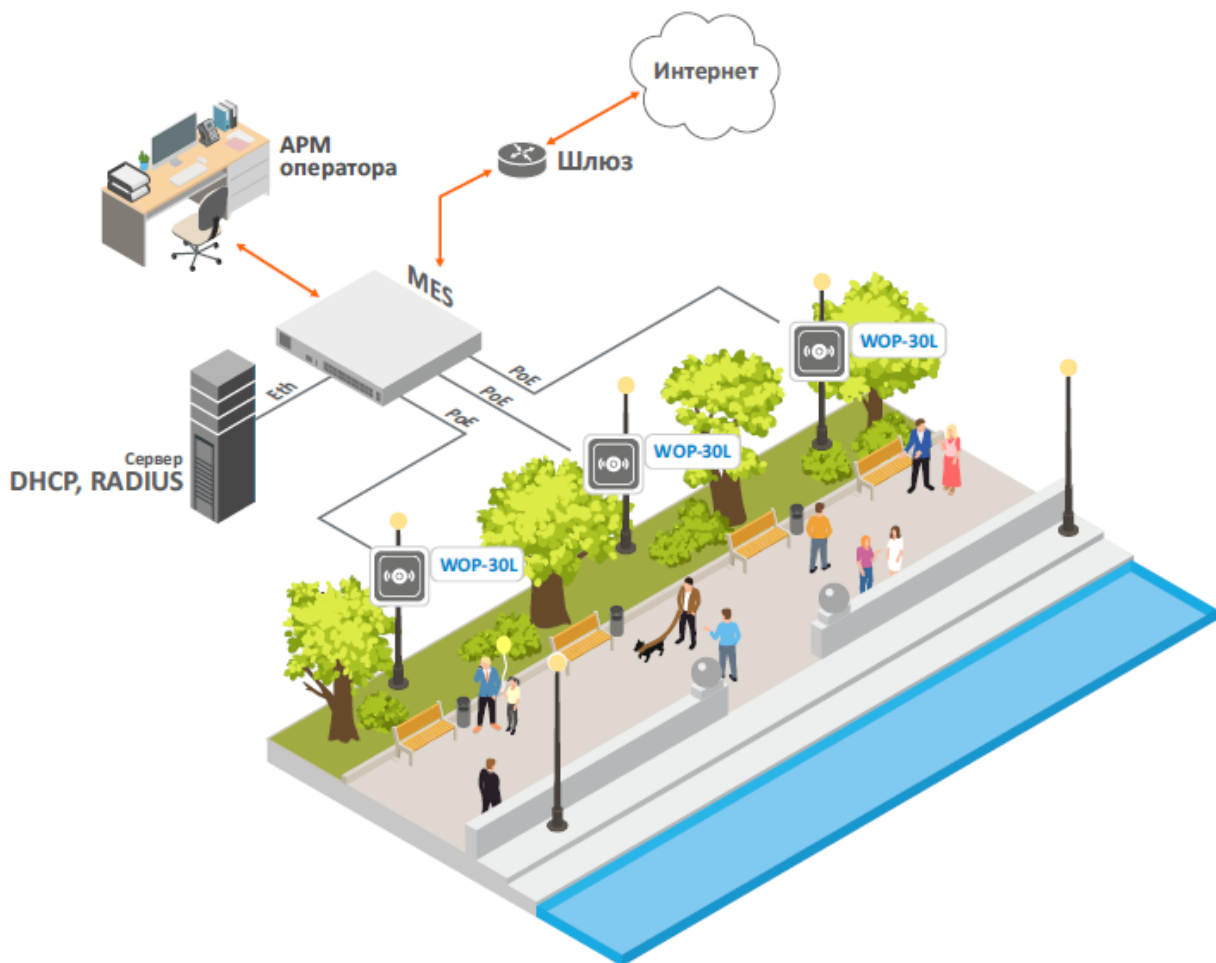
Рисунок 1 – Функциональная схема использования WOP-30L
