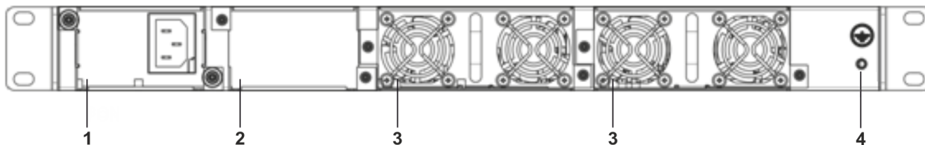
Рисунок 19 – Задняя панель ESR-1000
