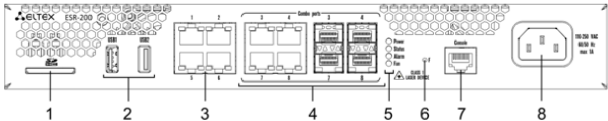
Рисунок 22 – Передняя панель ESR-200
