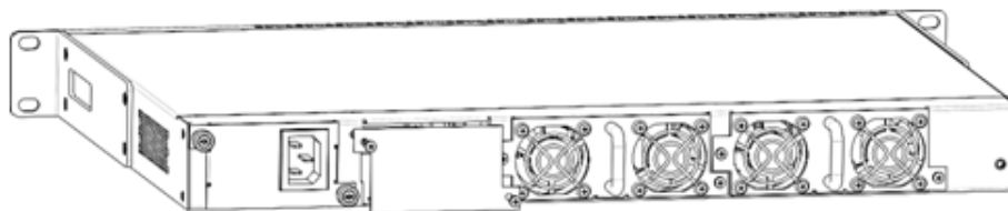
Рисунок 61 – Установка заглушки
