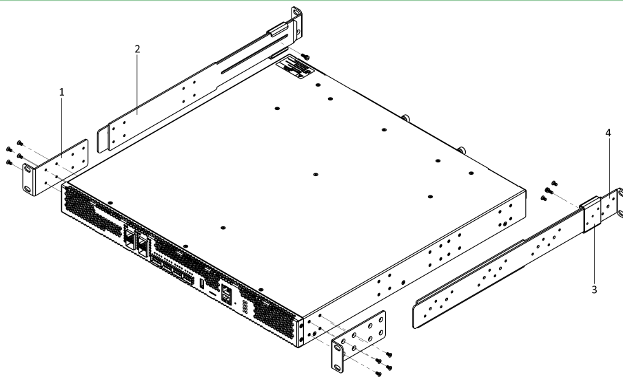
Рисунок 58 – Крепление кронштейнов к ESR-3300
