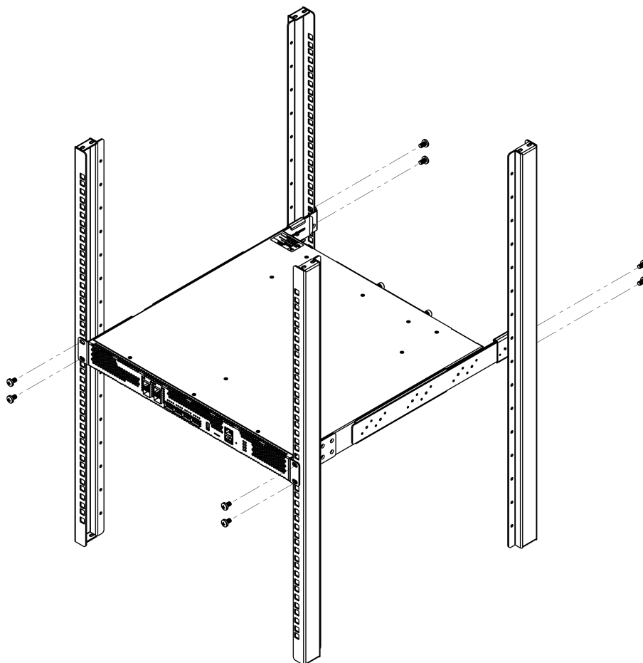
Рисунок 59 – Установка ESR-3300 в стойку
