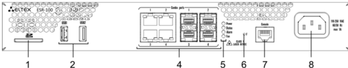
Рисунок 23 – Передняя панель ESR-100
