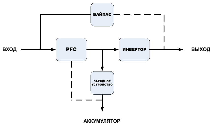
Рисунок 1-4. Нормальный режим
