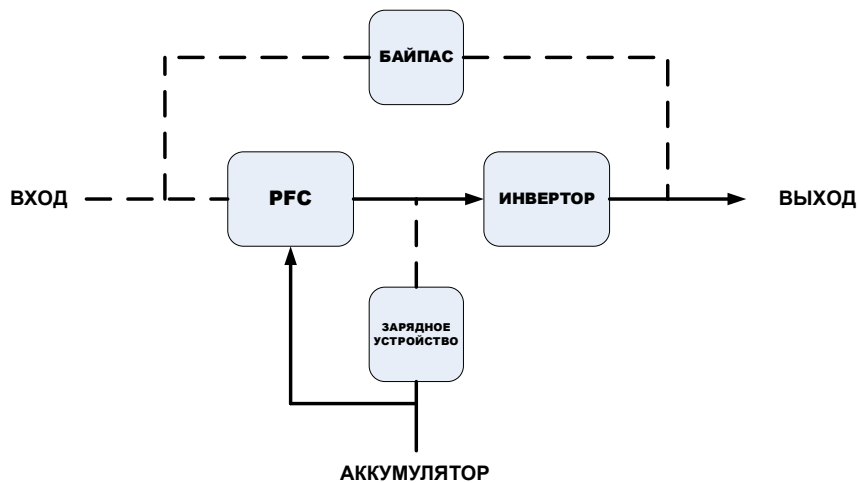
Рисунок 1-6. Режим аккумулятора
