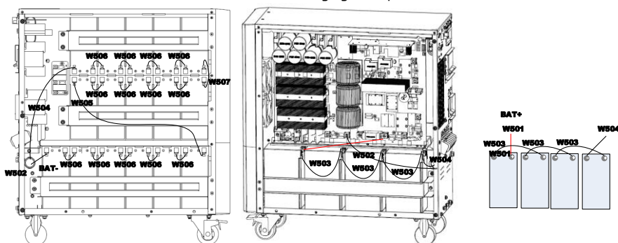
16 блоков аккумуляторов
