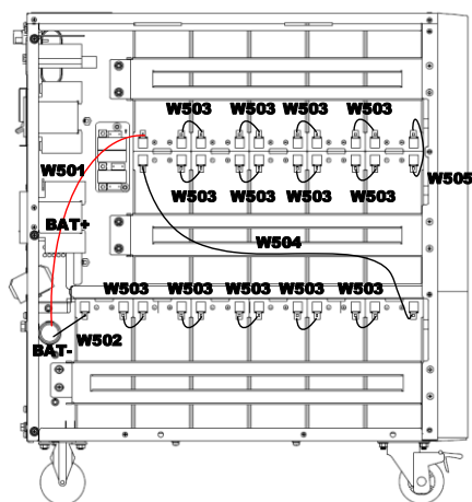
16 блоков аккумуляторов
