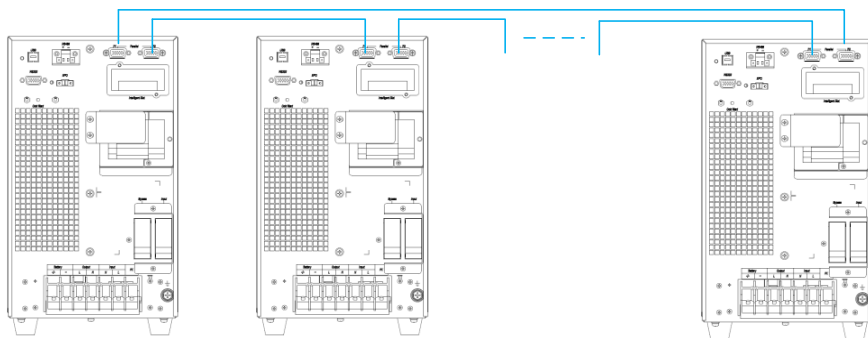
Рисунок 2-8. Система с 3 параллельно подключенными ИБП
