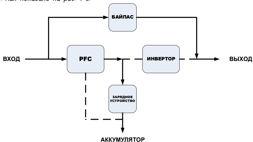
Рисунок 1-5. Режим байпаса
