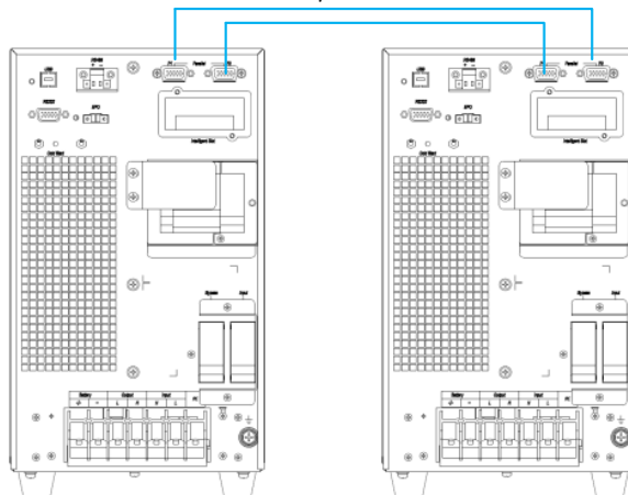
Рисунок 2-7. Система с 2 параллельно подключенными ИБП
