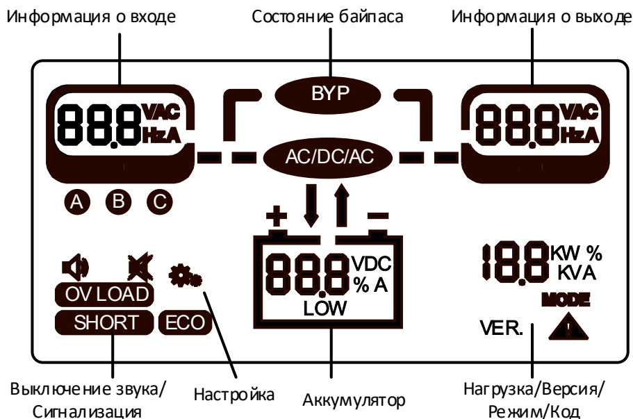
Рисунок 3-1. Меню ЖК-дисплея
