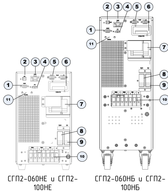
Рисунок 1-2. Вид сзади
