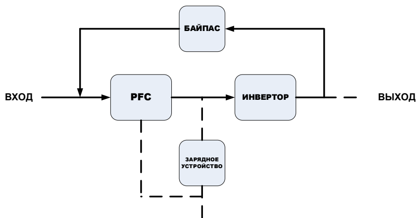
Рисунок 1-8. Режим самостарения
