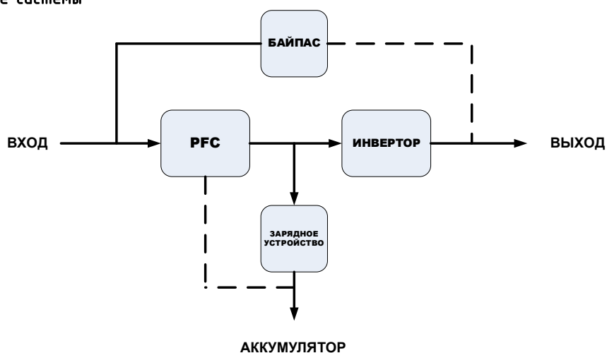
Рисунок 1-3. Система ИБП
