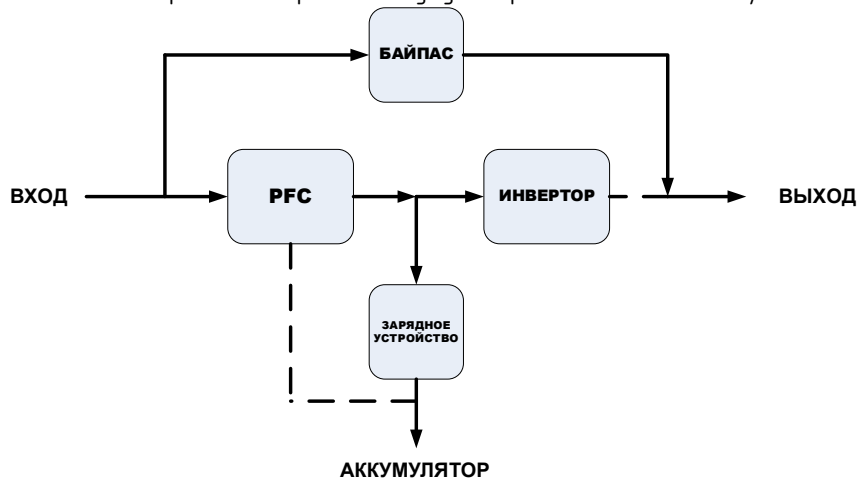
Рисунок 1-7. Режим ECO
