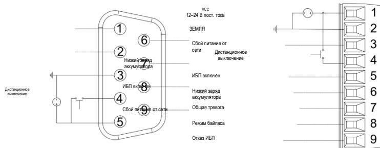
Рисунок 5-1. Сухой контакт
