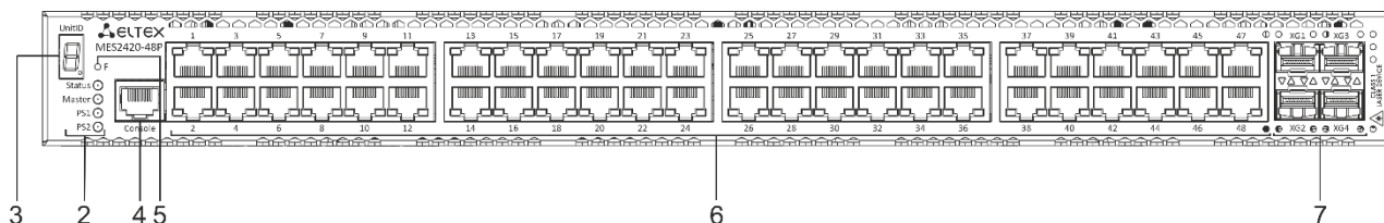
Рисунок 24 – Передняя панель MES2420-48P
