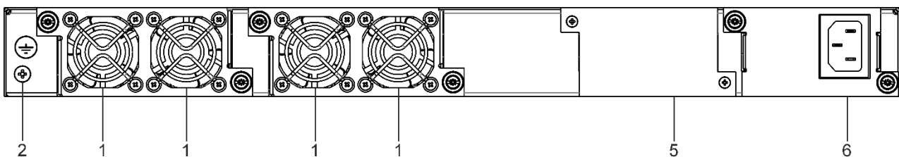
Рисунок 45 — Задняя панель MES3400-24, MES3400I-24, MES3400-48, MES3400-48F
