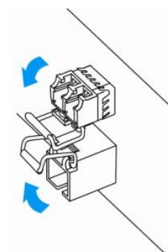
Рисунок 61 – Открытие защелки SFP-трансиверов
