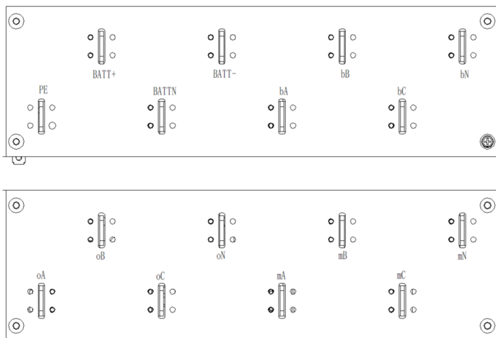
(с) Схема подключения клемм 10-слотового ИБП
