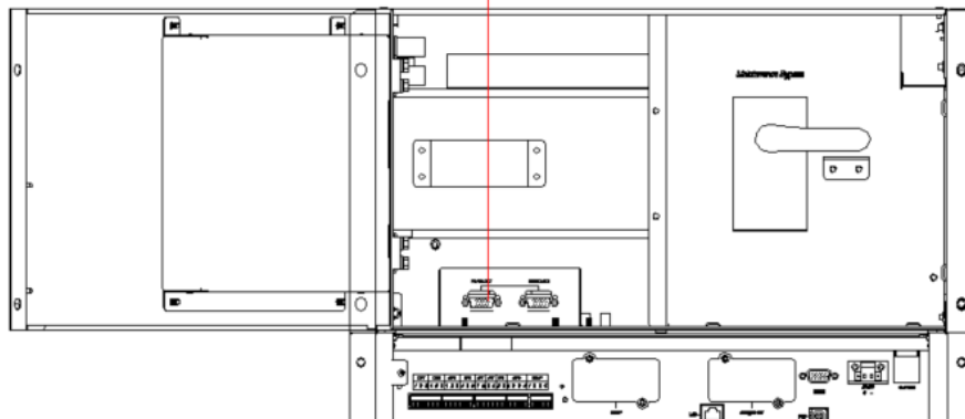
(а) Расположение порта параллельного подключения на 4- и 6-слотовых ИБП
