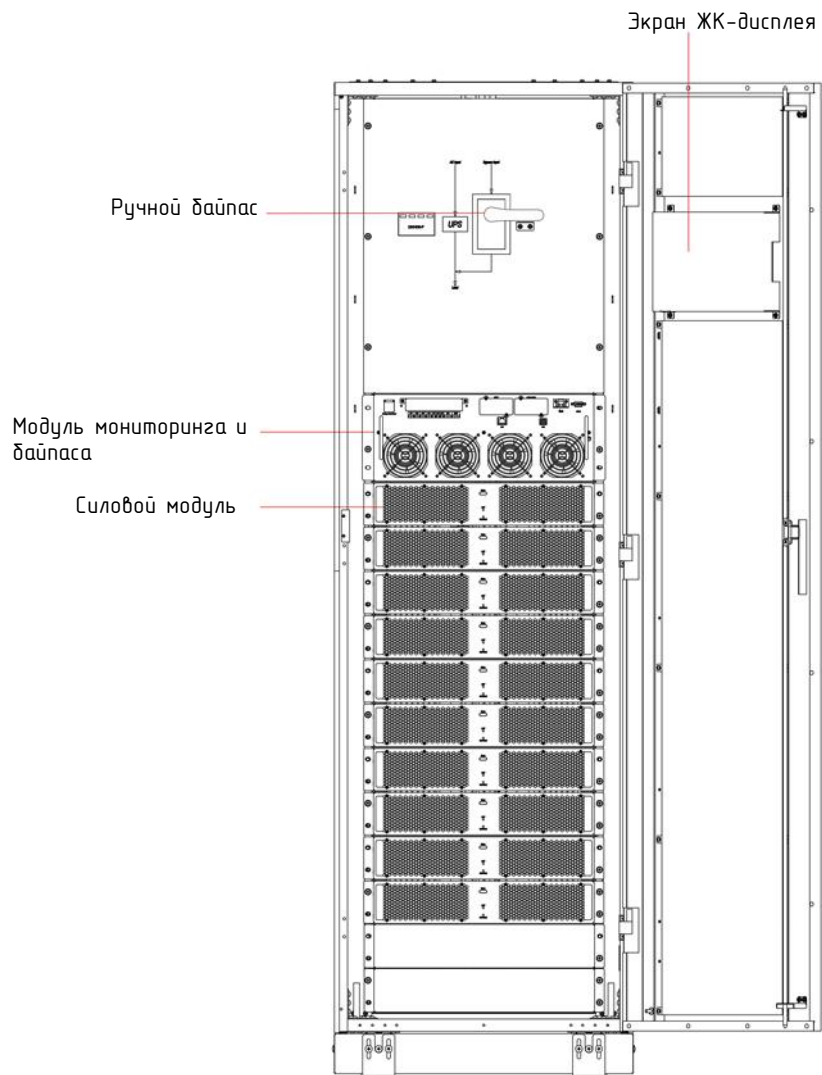
(с) Вид спереди 10-слотового ИБП Рисунок 2-8. Вид системы спереди
