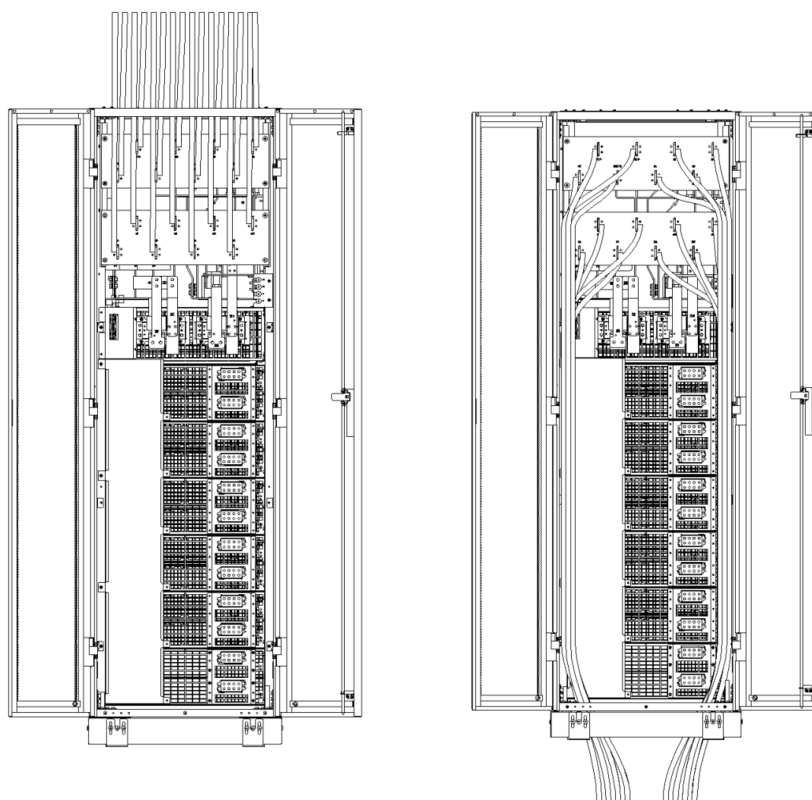
(б) Схема ввода кабелей снизу для 10-слотового ИБП Рисунок 3-11. Схема ввода кабелей
