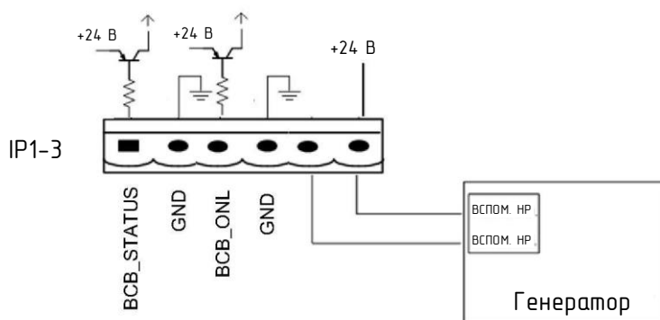
Рисунок 3-13. Схема входного порта для входа генератора
