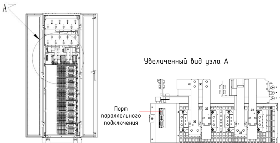
(б) Расположение порта параллельного подключения на 10-слотовом ИБП
