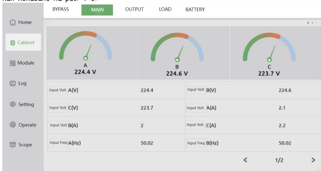
Рисунок 4-5. Меню Cabinet (Блок)
