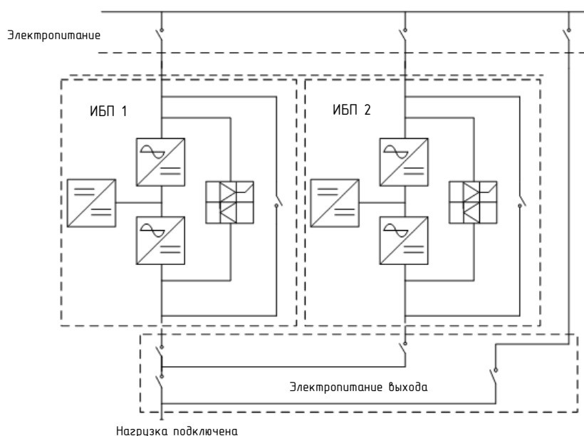
Рисунок 5-5. Структура параллельного подключения
