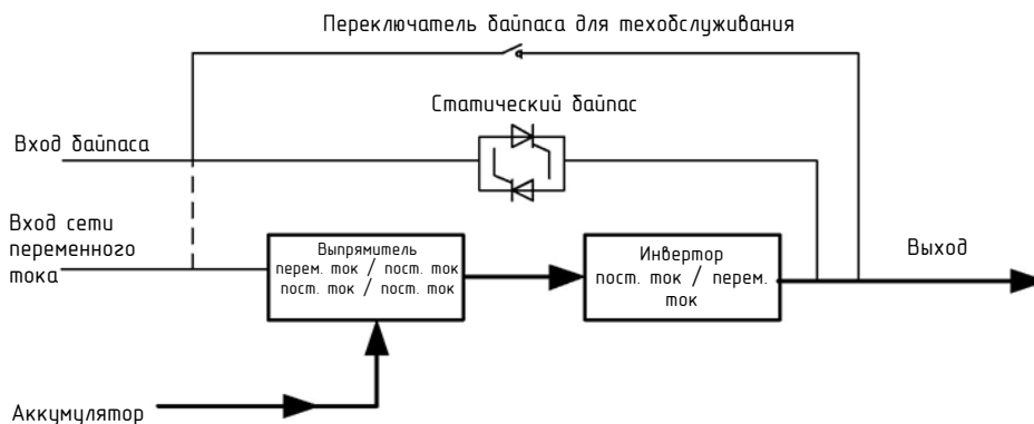
Рисунок 2-4. Схема режима работы от аккумуляторов
