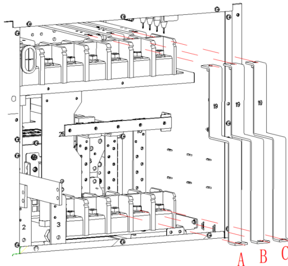
(а) Схема короткой медной шины, соединяющей вход сети переменного тока с входом байпаса 4-слотового и 6-слотового ИБП
