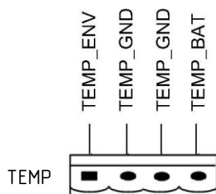
Рисунок 3-12. TEMP 1-4 для контроля температуры
