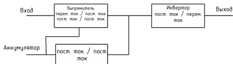
Рисунок 2-2. Схема силового модуля
