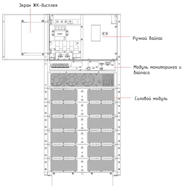
(б) Вид спереди 6-слотового ИБП
