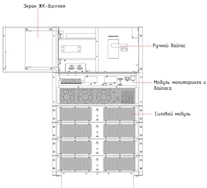
(а) Вид спереди 4-слотового ИБП
