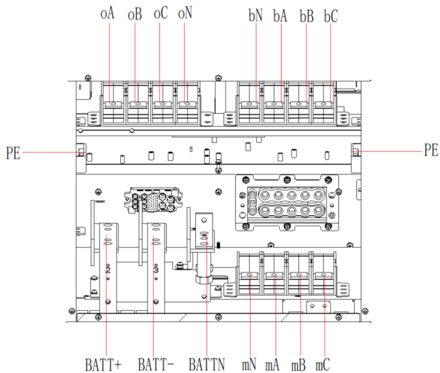
(a) Схема подключения клемм 4-слотового ИБП
