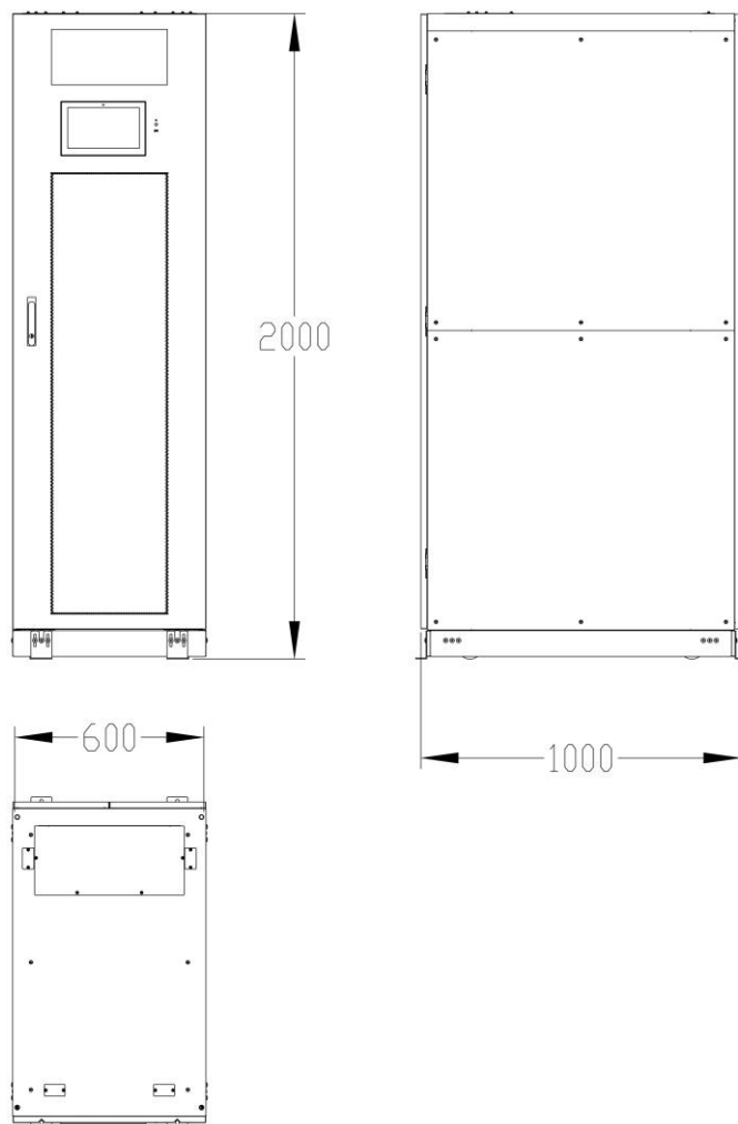
(с) Габаритная схема 10-слотового ИБП (ед. изм.: мм) Рисунок 3-1. Габаритная схема ИБП (ед. изм.: мм)
