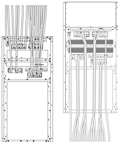
(а) Схема ввода кабелей сверху для 4-слотового и 6-слотового ИБП
