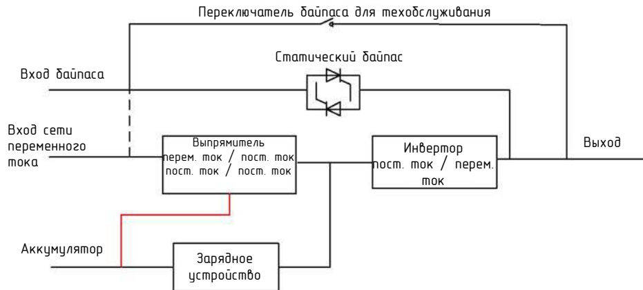
Рисунок 2-1. Схема ИБП
