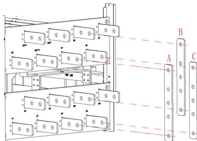
(б) Схема короткой медной шины, соединяющей вход сети переменного тока с входом байпаса 10-слотового ИБП
