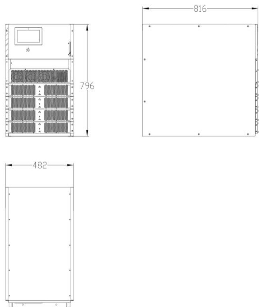
(а) Габаритная схема 4-слотового ИБП (ед. изм.: мм)
