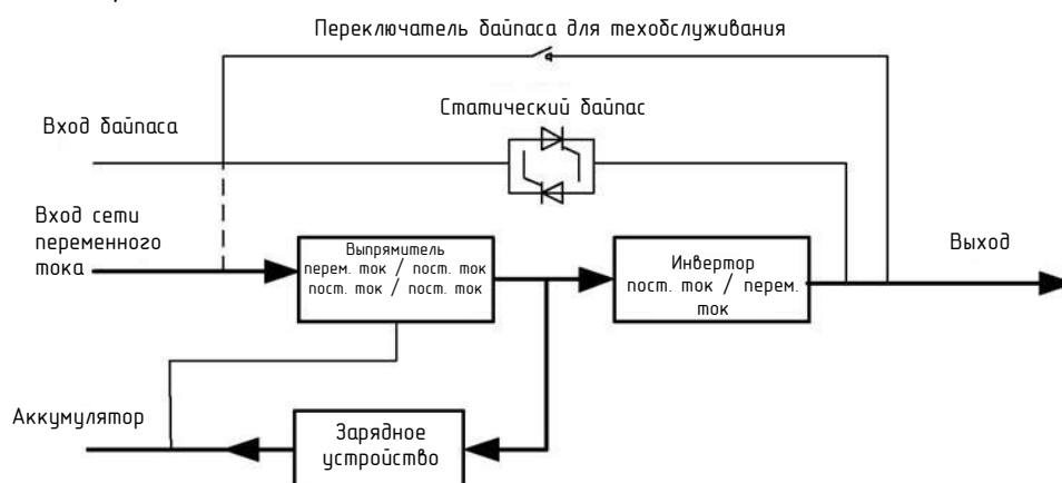
Рисунок 2-3. Схема нормального режима работы
