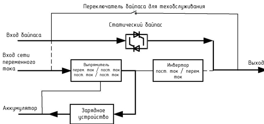
Рисунок 2-5. Схема режима байпаса
