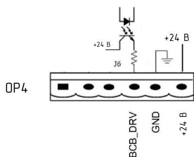
Рисунок 3-14. Порт АВ аккумулятора
