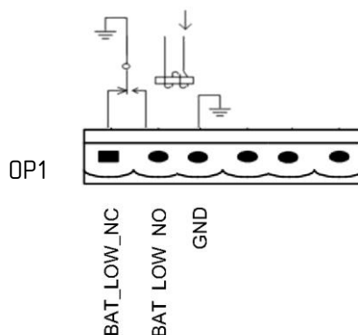
Рисунок 3-15. Схема интерфейса с сухим контактом выходного предупреждающего сигнала аккумуляторов
