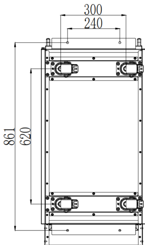
(b) 6-слотовый ИБП (вид снизу, ед. изм.: мм)
