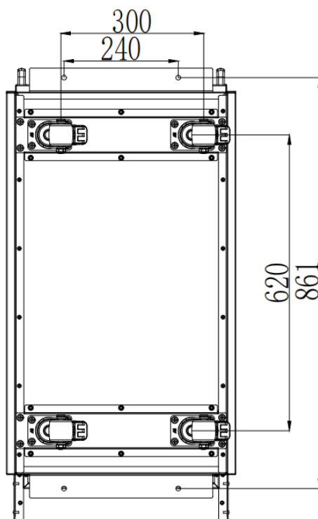
(а) 4-слотовый ИБП (вид снизу, ед. изм.: мм)
