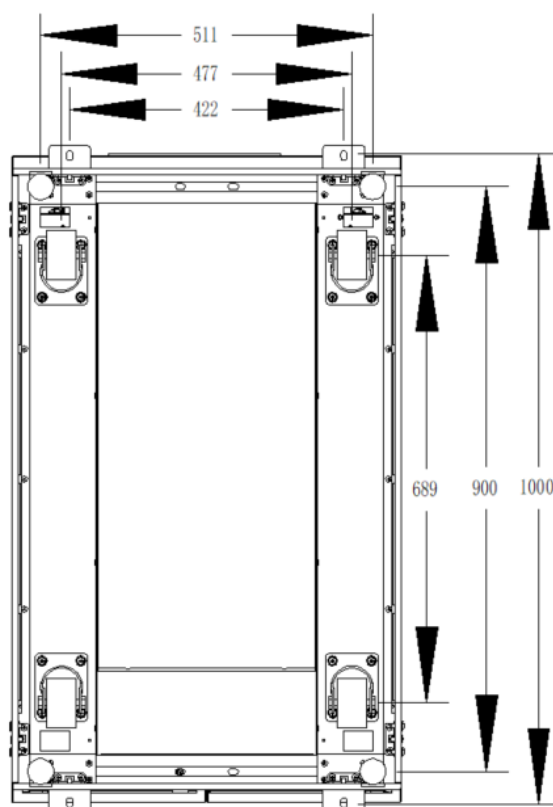
(c) 10-слотовый ИБП (вид снизу, ед. изм.: мм)
