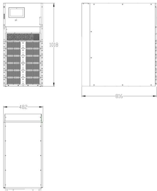
(б) Габаритная схема 6-слотового ИБП (ед. изм.: мм)
