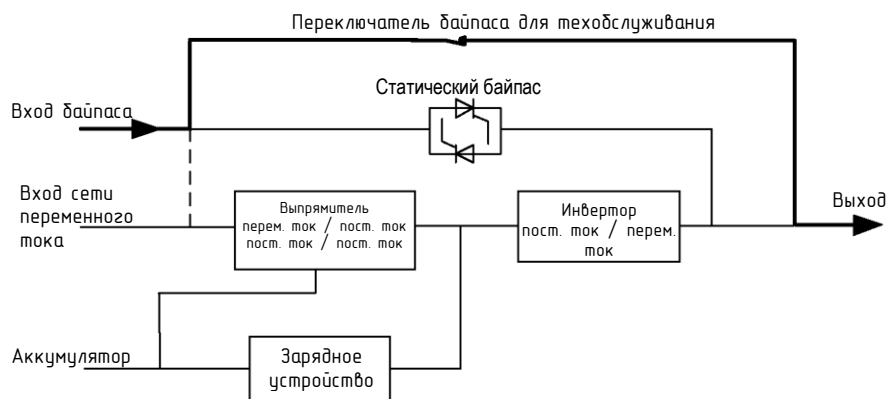
Рисунок 2-6. Схема режима техобслуживания
