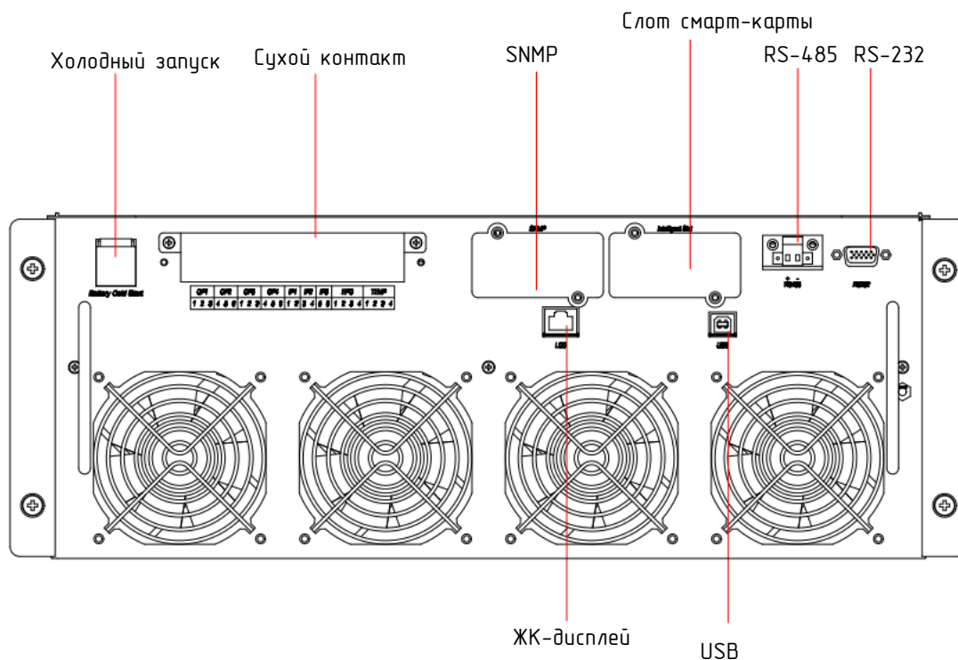
(б) Интерфейс связи для 10-слотового ИБП Рисунок 3-14. Схема интерфейса связи
