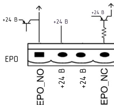
Рисунок 3-11. Схема порта входа дистанционного EPO
