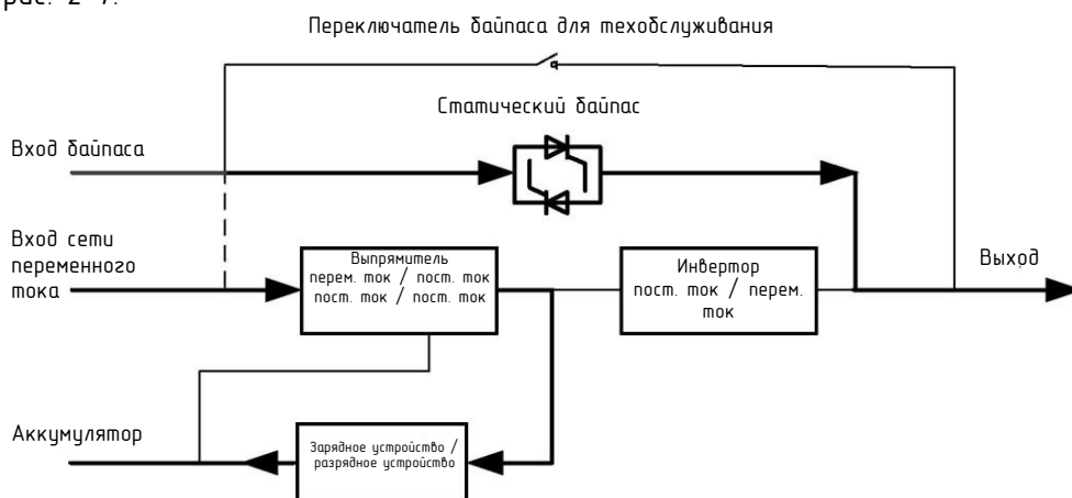
Рисунок 2-7. Схема работы в режиме ESO
