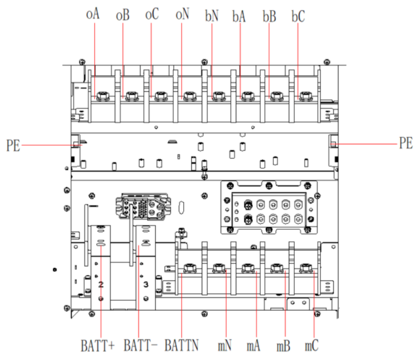
(b) Схема подключения клемм 6-слотового ИБП
