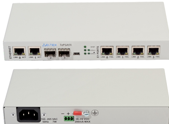
TopGATE-4E1-2FG
