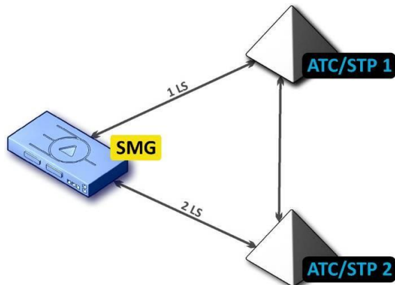
Рисунок 18 — Схема подключения SMG при работе в квазисвязанном режиме через АТС с STP (LS — группа линий ОКС-7 (Link Set))
