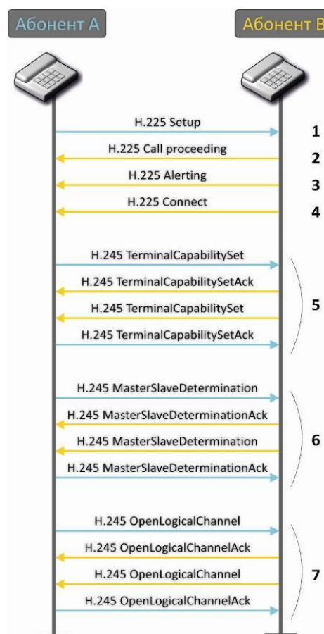
Рисунок 20 – Алгоритм вызова по протоколу H.323
