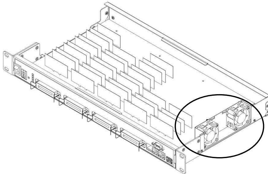
Рисунок 6 – Расположение вентиляторов
