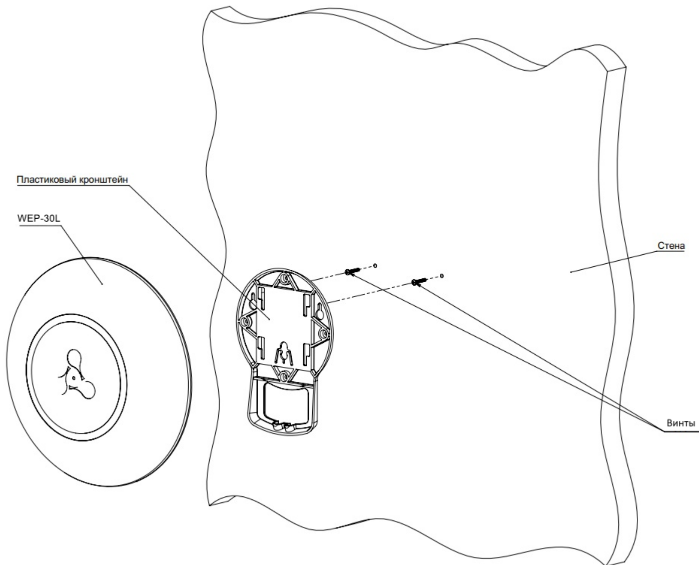
Рисунок 7 – Крепление кронштейна на стене
