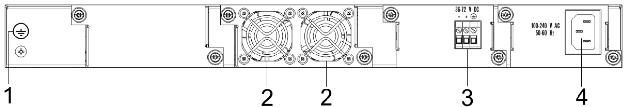
Рисунок 41 – Задняя панель MES5316A
