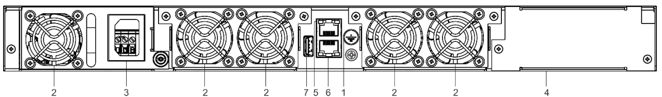
Рисунок 42 – Задняя панель MES5310-48
