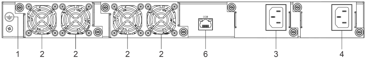
Рисунок 38 – Задняя панель MES3300-48, MES3300-48F
