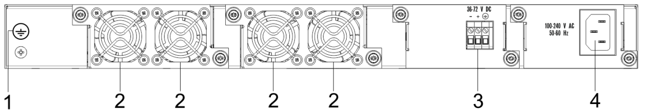
Рисунок 40 – Задняя панель MES5312, MES5324A, MES5332A
