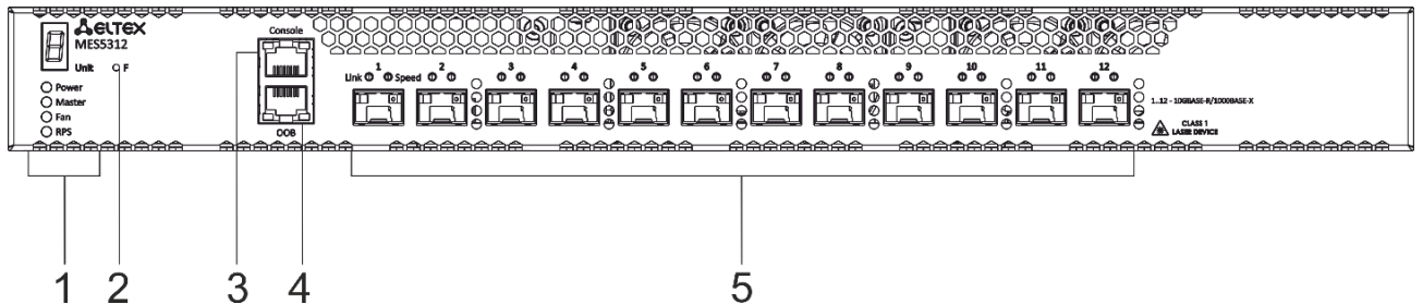
Рисунок 16 – Передняя панель MES5312
