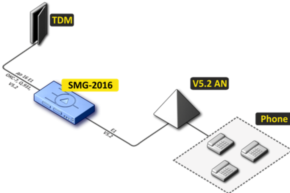
Рисунок 7 – Вынос V5.2 AN на базе SMG-2016
