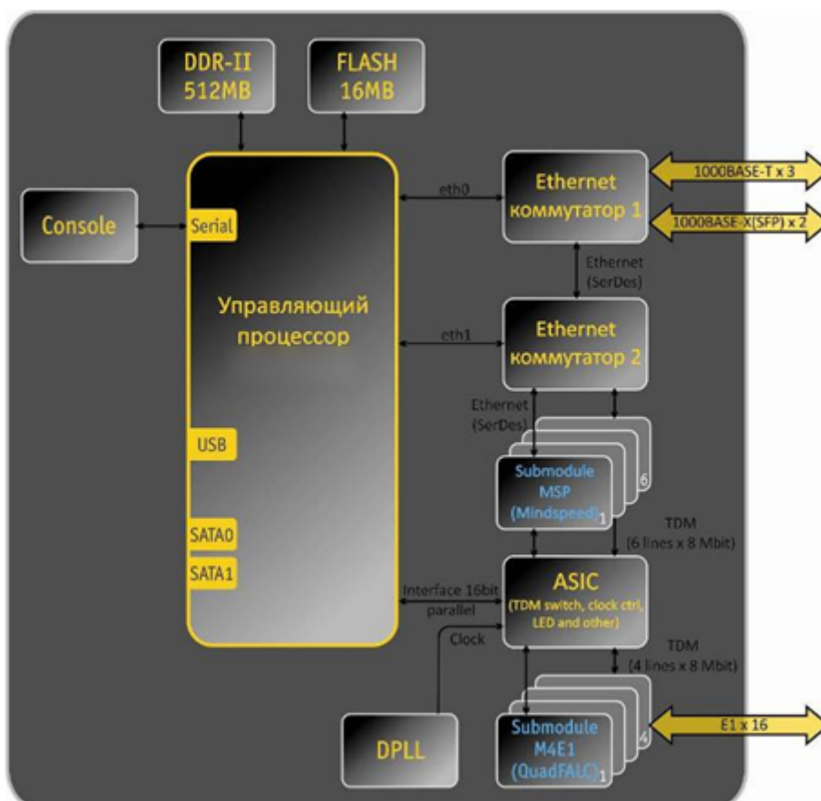
Рисунок 9 – Функциональная схема SMG-1016M
