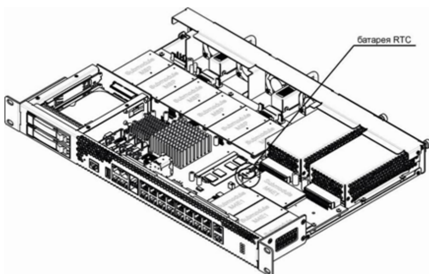
Рисунок 43 – Положение батареи RTC для SMG-2016
