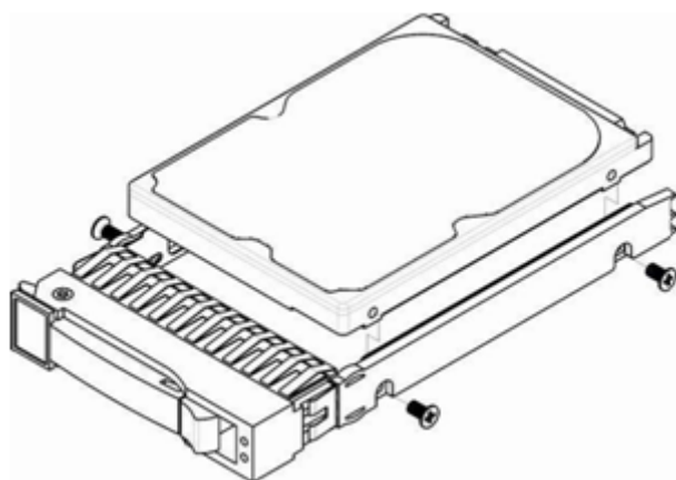
Рисунок 40 – Крепление SATA-диска в лоток направляющих салазок
