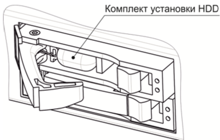
Рисунок 39 – Расположение комплекта крепежных элементов при поставке
