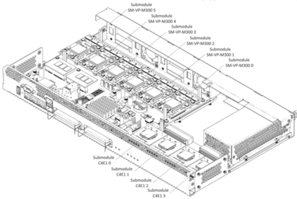
Рисунок 27 – Расположение субмодулей в SMG-1016M
