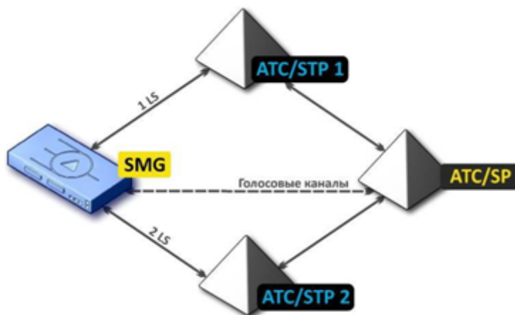
Рисунок 48 – Схема подключения SMG в комбинированном режиме
