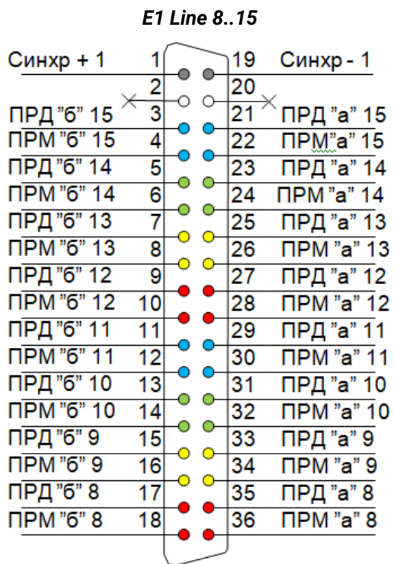
Рисунок 50 – Назначение контактов разъемов E1 Line
