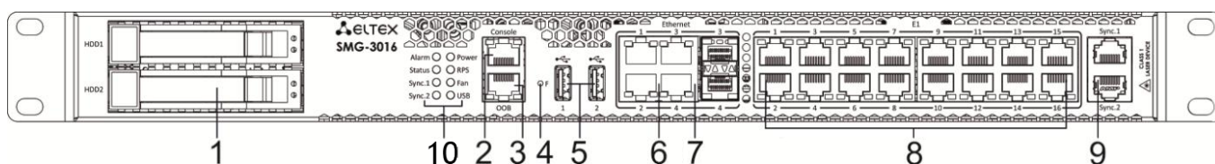
Рисунок 17 – Внешний вид передней панели SMG-3016
