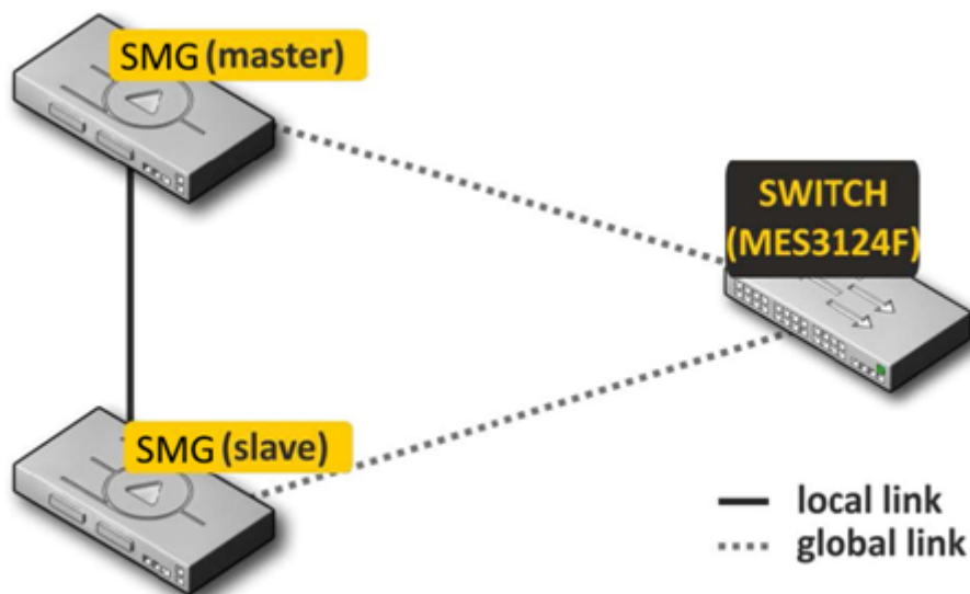
Рисунок 54 – Схема резервирования с одним коммутатором
