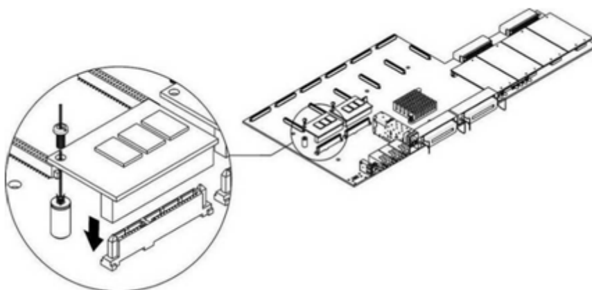
Рисунок 38 – Монтаж SSD-накопителя
