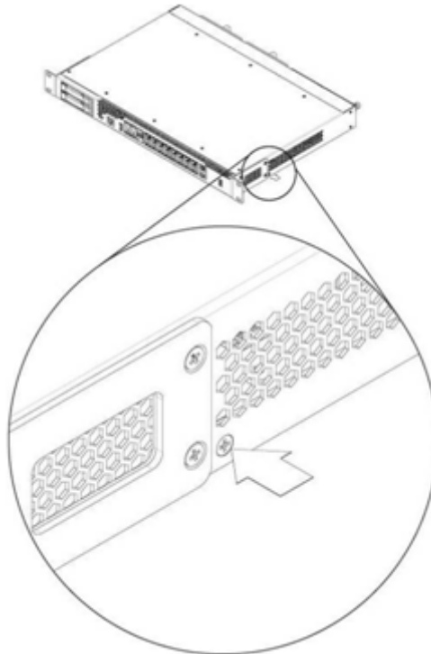
Рисунок 26 – Сборка SMG в корпус
