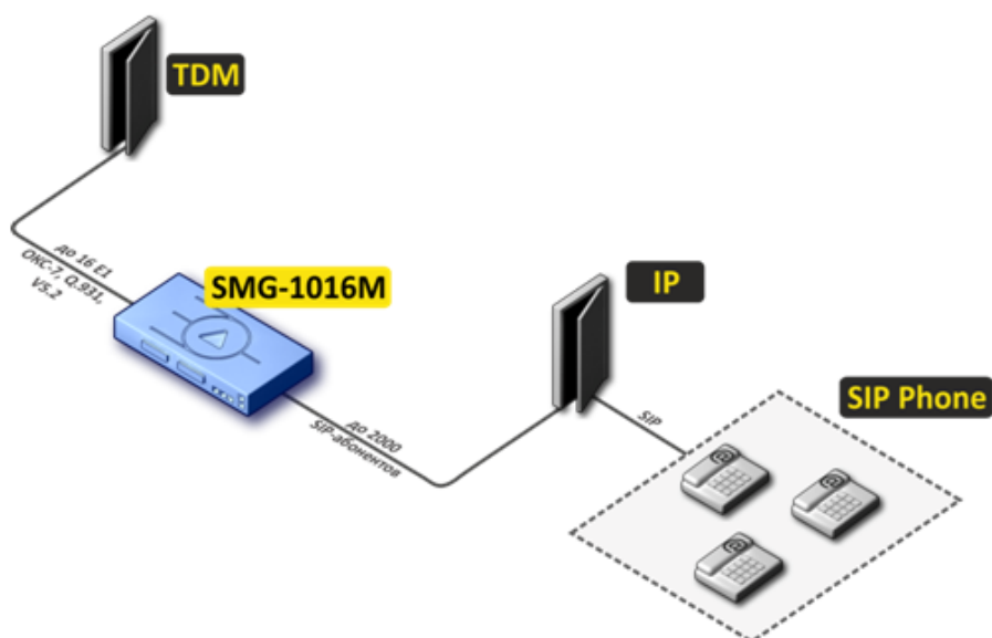
Рисунок 3 – Мини IP-PBX на базе SMG-1016M
