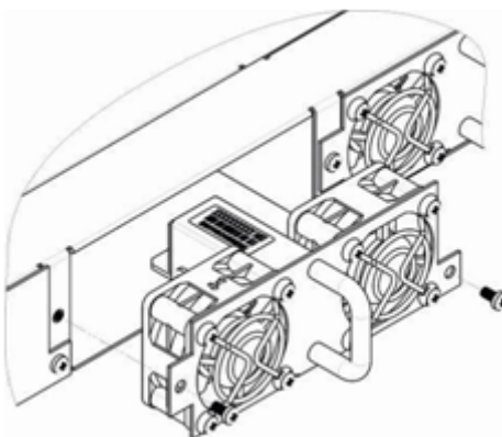
Рисунок 33 – Блок вентиляции SMG-2016. Крепление в корпус
