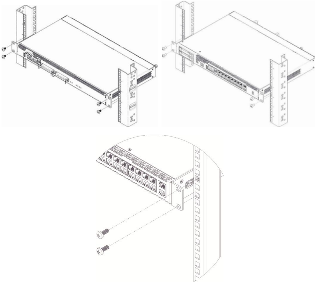
Рисунок 20 – Установка устройства в стойку SMG-1016M (слева), SMG-2016 (справа) и SMG-3016 (внизу)
