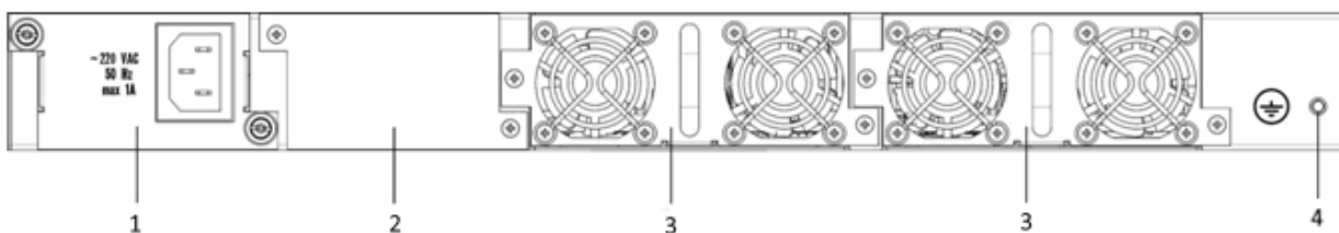
Рисунок 16 – Внешний вид задней панели SMG-2016
