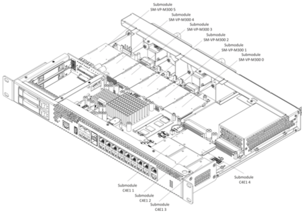
Рисунок 28 – Расположение субмодулей в SMG-2016
