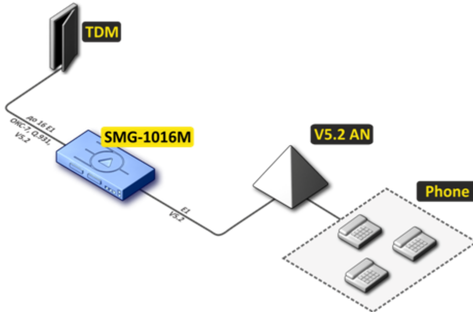
Рисунок 6 – Вынос V5.2 AN на базе SMG-1016M
