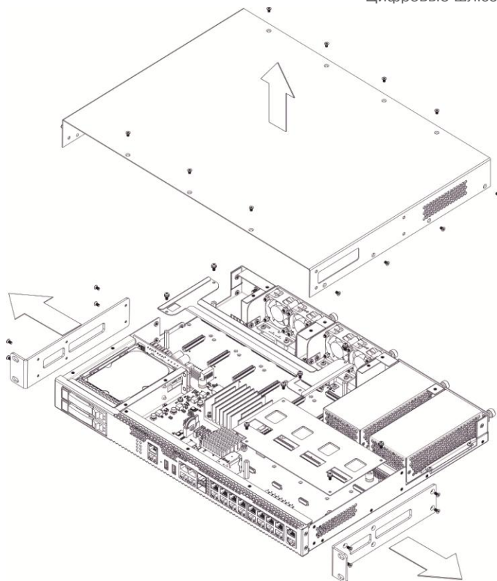
Рисунок 24 – Порядок вскрытия корпуса SMG-3016
