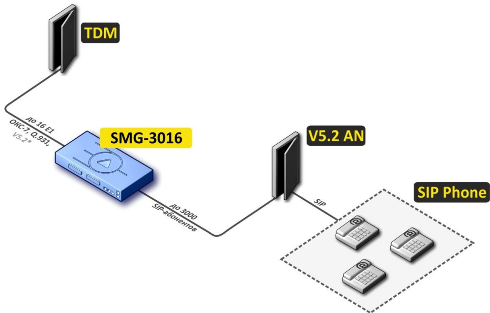
Рисунок 8 – Вынос V5.2 AN на базе SMG-3016
