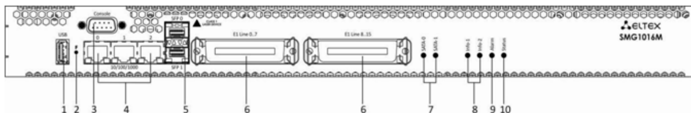
Рисунок 13 – Внешний вид передней панели SMG-1016M
