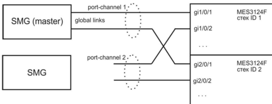
Рисунок 57 – Схема подключения ведущей SMG (master)
