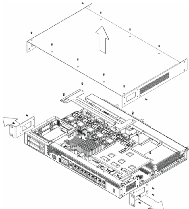
Рисунок 23 – Порядок вскрытия корпуса SMG-2016
