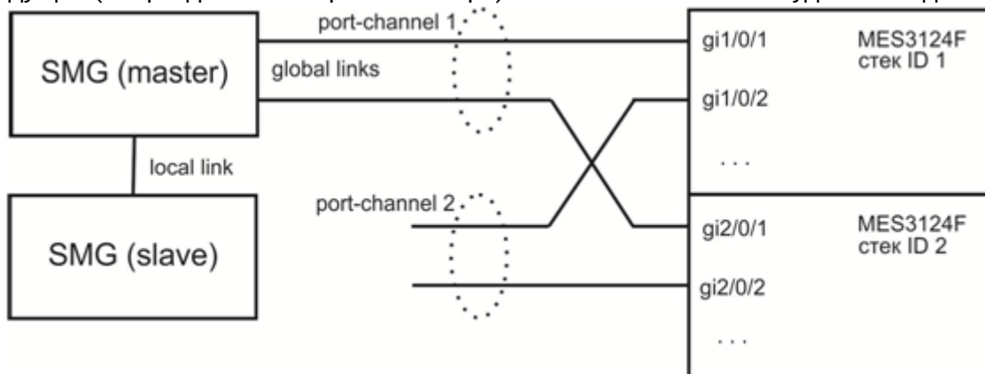
Рисунок 58 – Схема подключения ведомого SMG (slave)
