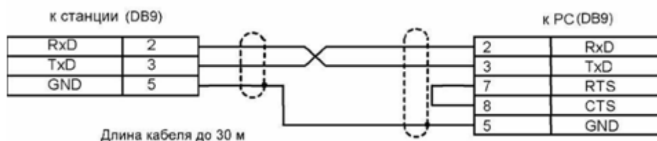
Рисунок 52 – Схема кабеля для подключения к ПОРТ1, ПОРТ2
