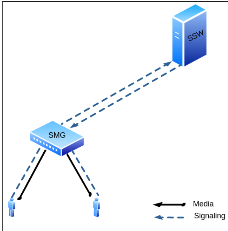
Рисунок 2 – MSR расположен на SMG
