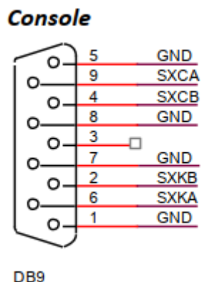
Рисунок 51 – Назначение контактов разъема Console
