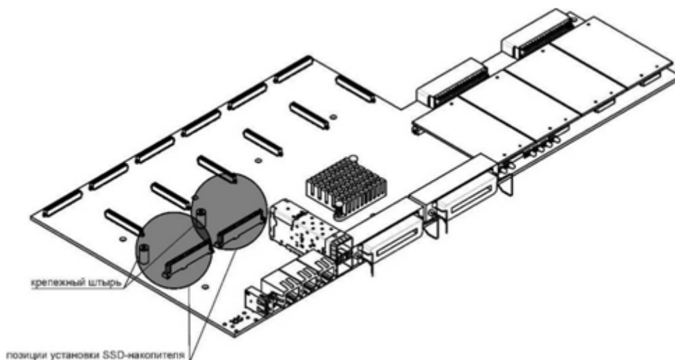
Рисунок 37 – Установка SSD-накопителя
