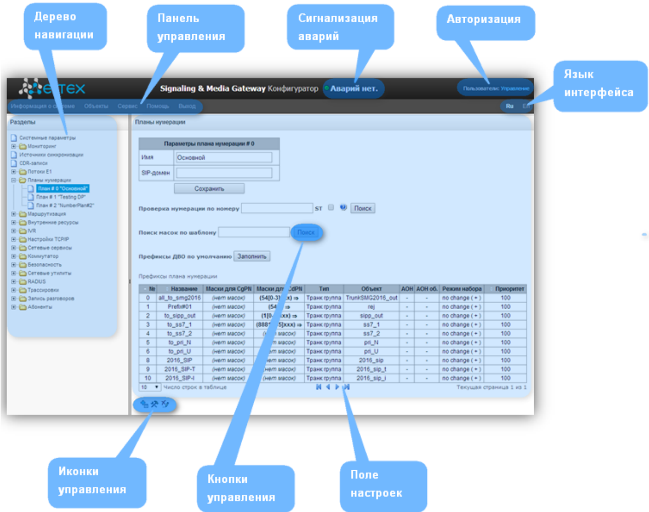
Рисунок 45 – Элементы навигации web-конфигуратора
