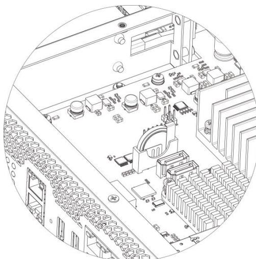
Рисунок 44 – Положение батареи RTC для SMG-3016
