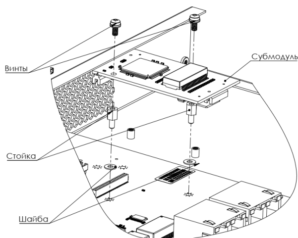
Рисунок 30 – Установка субмодуля на плату
