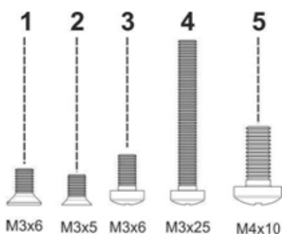
Рисунок 25 – Типы винтов для сборки SMG
