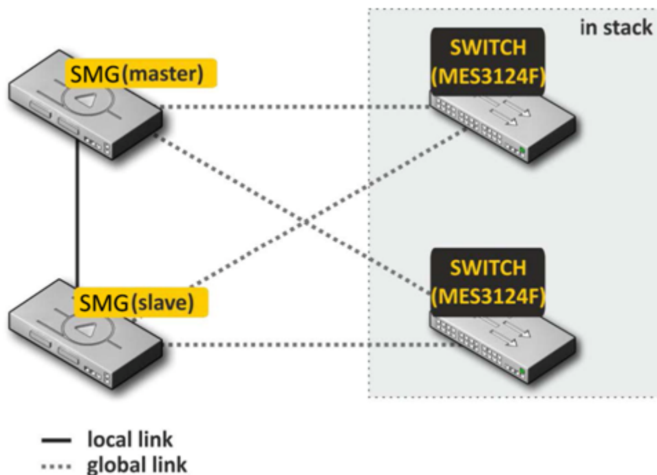
Рисунок 55 – Схема резервирования двумя коммутаторами в стеке
