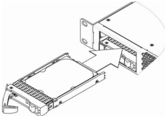
Рисунок 41 – Монтаж SATA-диска в корпус устройства
