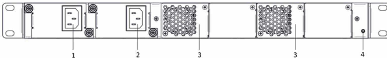
Рисунок 14 – Внешний вид задней панели SMG-1016M
