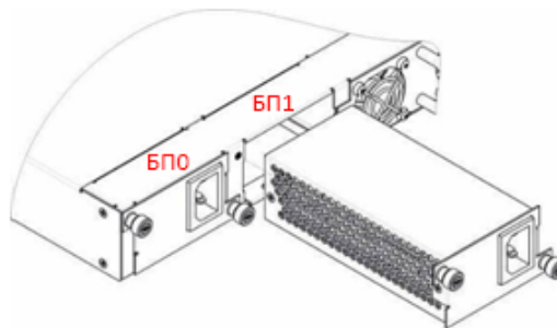
Рисунок 21 – Установка модулей питания
