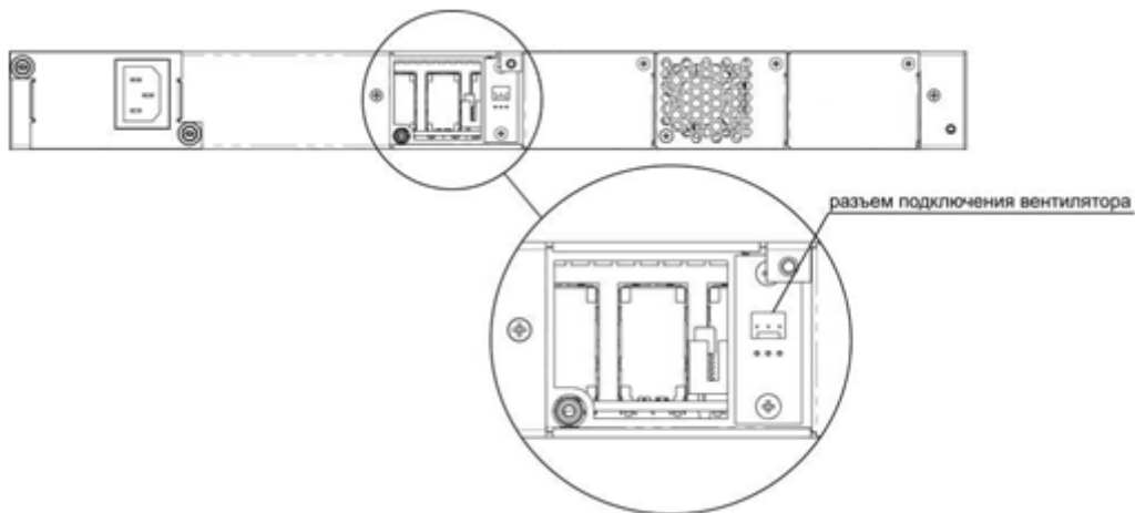
Рисунок 36 – Разъем для подключения вентилятора
