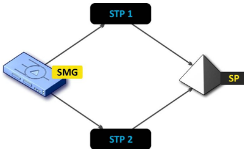
Рисунок 46 – Схема подключения SMG при работе в квазисвязанном режиме через STP
