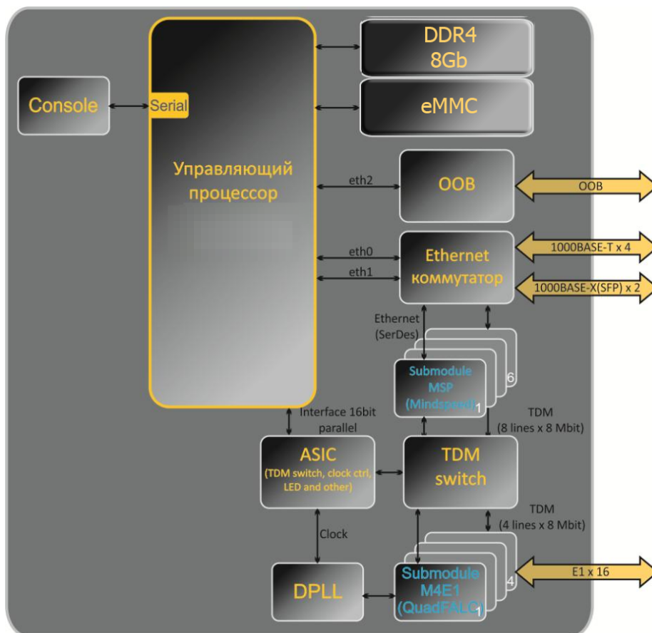
Рисунок 11 – Функциональная схема SMG-3016
