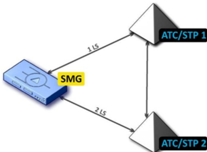
Рисунок 47 – Схема подключения SMG при работе в квазисвязанном режиме через АТС с STP (LS – группа линий ОКС-7 (Link Set))
