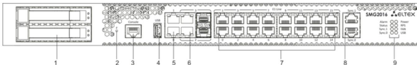
Рисунок 15 – Внешний вид передней панели SMG-2016
