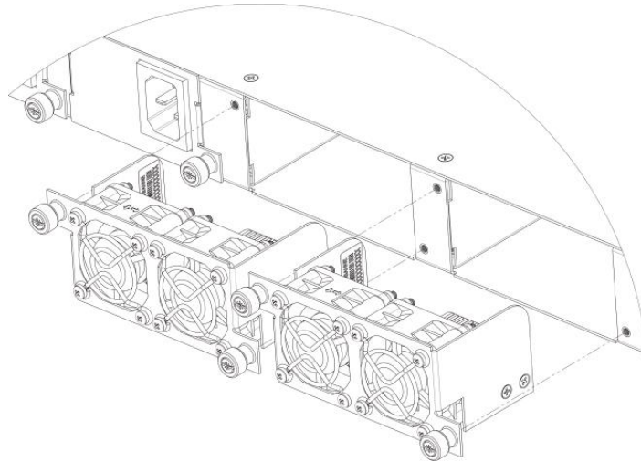
Рисунок 35 – Блок вентиляции SMG-3016. Крепление в корпус
