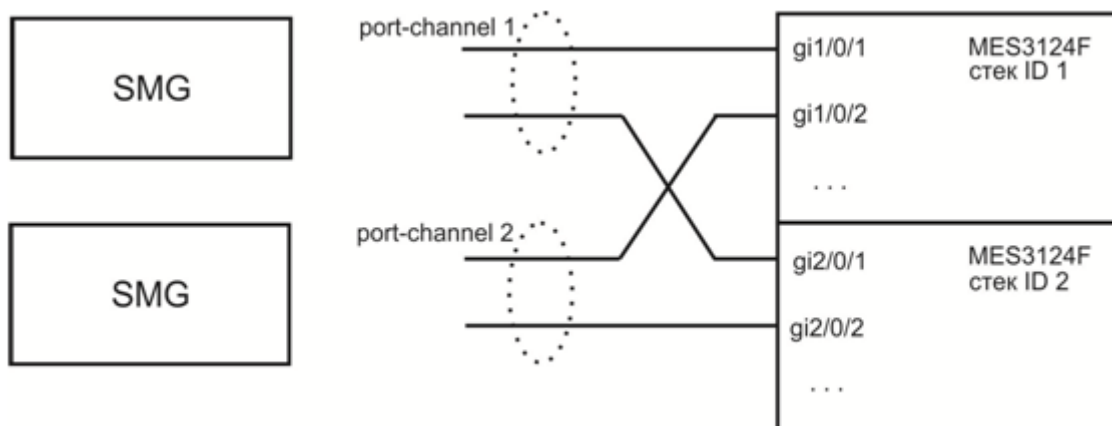
Рисунок 56 – Схема объединения портов в port-channel
