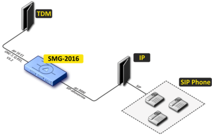
Рисунок 4 – Мини IP-PBX на базе SMG-2016
