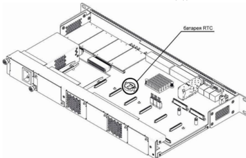
Рисунок 42 – Положение батареи RTC для SMG-1016M
