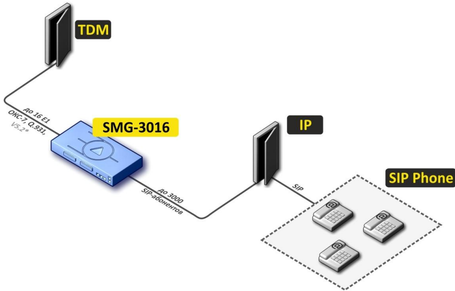
Рисунок 5 – Мини IP-PBX на базе SMG-3016
