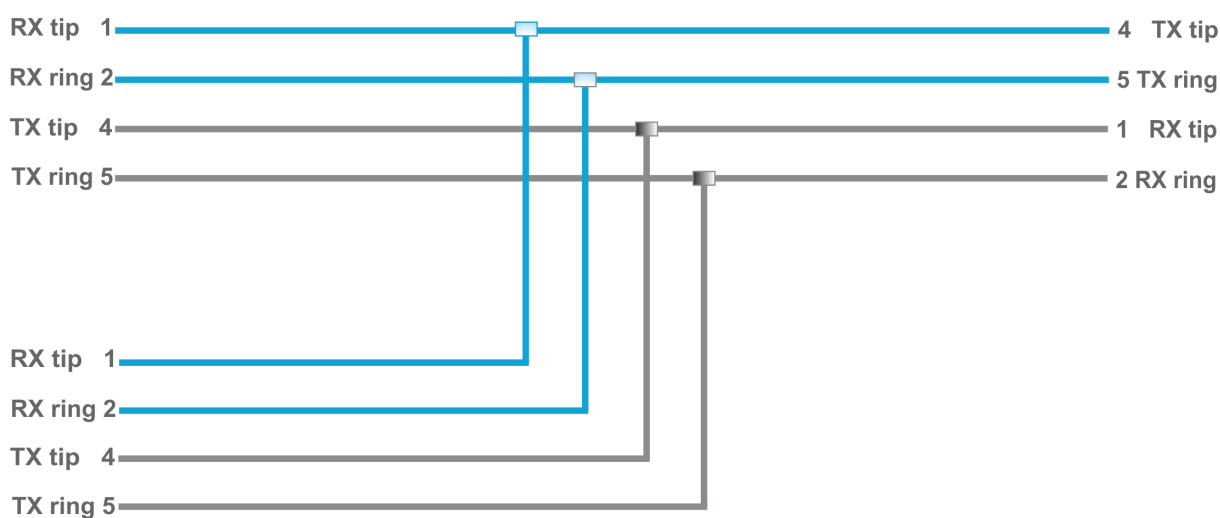
Схема распайки кабеля для резервирования E1
