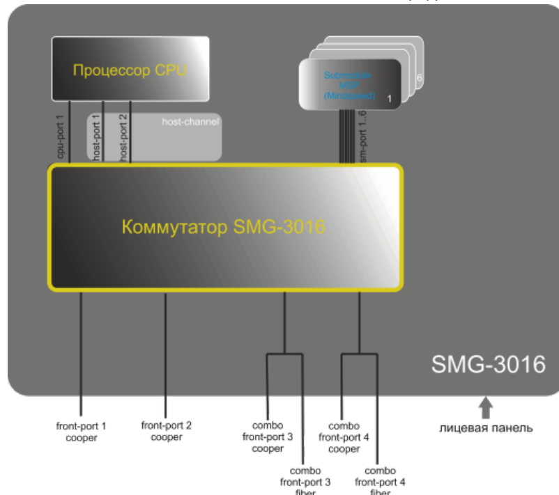
Рисунок 49 – Структура коммутатора
