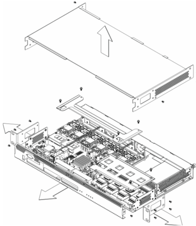
Рисунок 22 – Порядок вскрытия корпуса SMG-1016M
