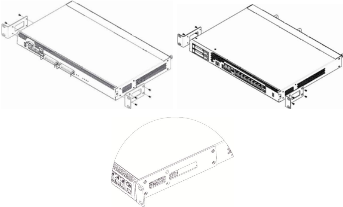
Рисунок 19 – Крепление кронштейнов для SMG-1016M (сверху слева), SMG-2016 (сверху справа) и SMG-3016 (внизу)
