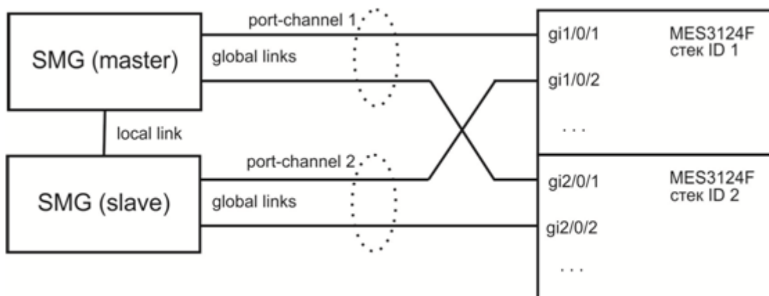
Рисунок 59 – Схема подключения global links
