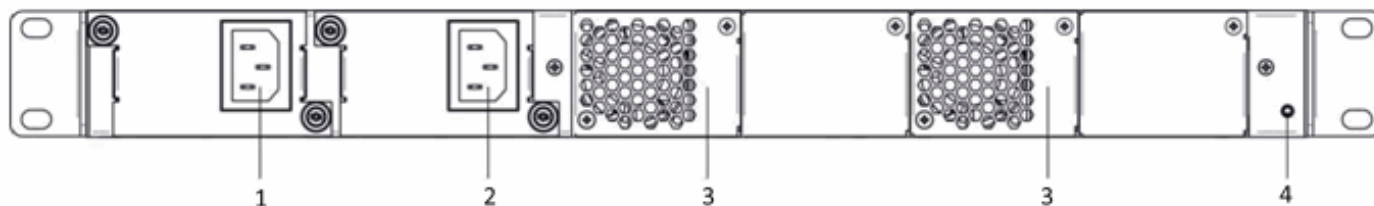
Рисунок 18 – Внешний вид задней панели SMG-3016
