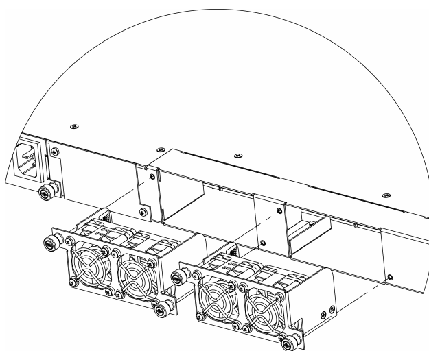
Рисунок 34 – Блок вентиляции SMG-2016 rev. B. Крепление в корпус
