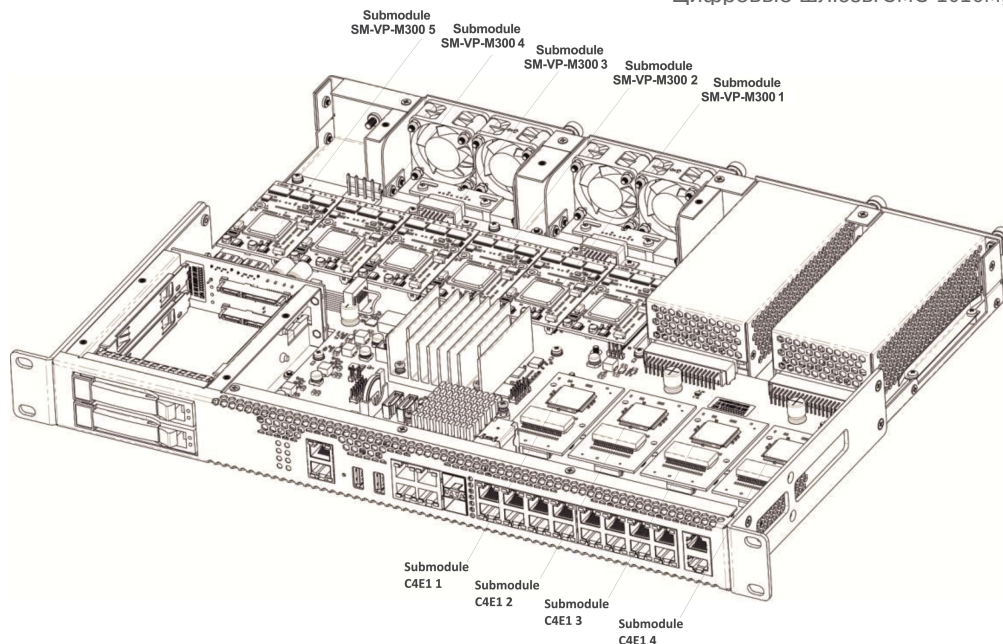
Рисунок 29 – Расположение субмодулей в SMG-3016
