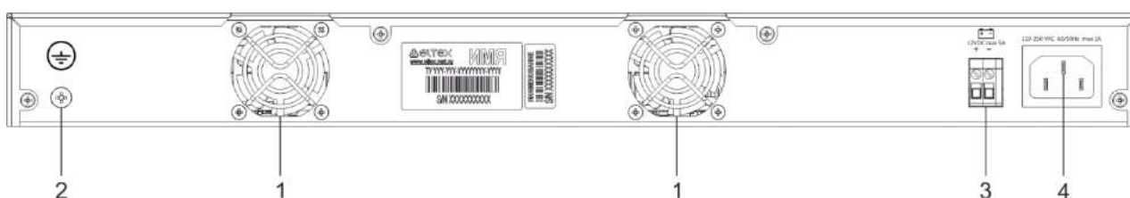
Рисунок 30 – Задняя панель MES2448B
