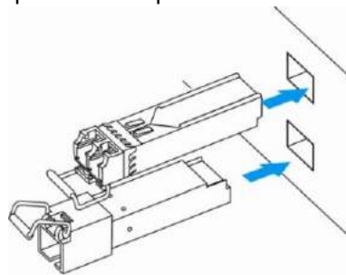
Рисунок 43 – Установка SFP-трансиверов
