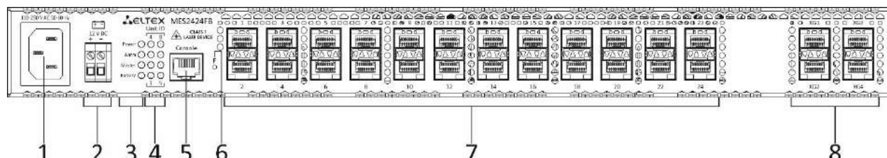
Рисунок 24 — Передняя панель MES2424FB
