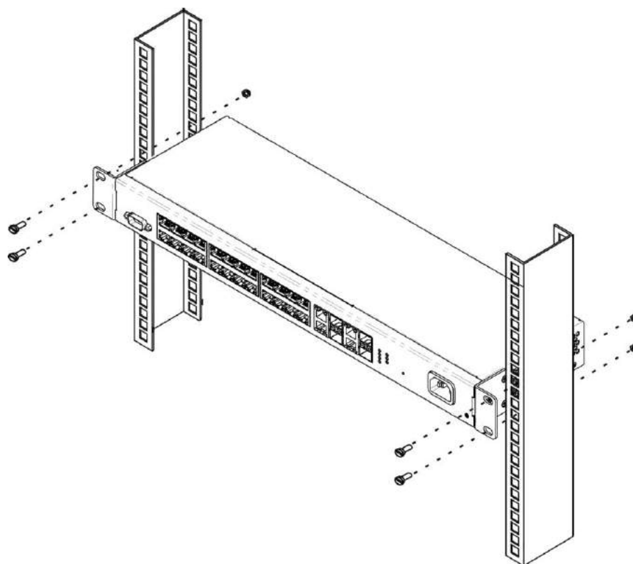
Рисунок 41 – Установка устройства в стойку
