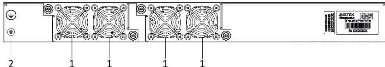
Рисунок 33 – Задняя панель MES2424FB
