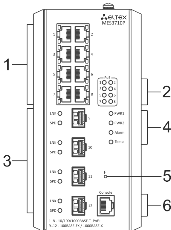
Рисунок 25 – Передняя панель MES3710P
