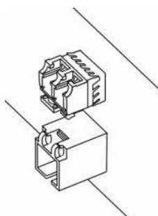
Рисунок 44 – Установленные SFP-трансиверы
