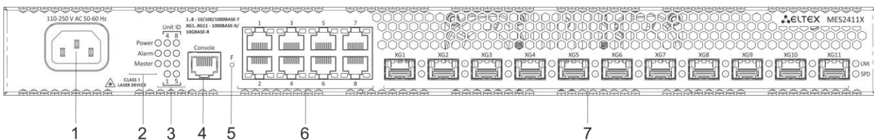
Рисунок 23 – Передняя панель MES2411X
