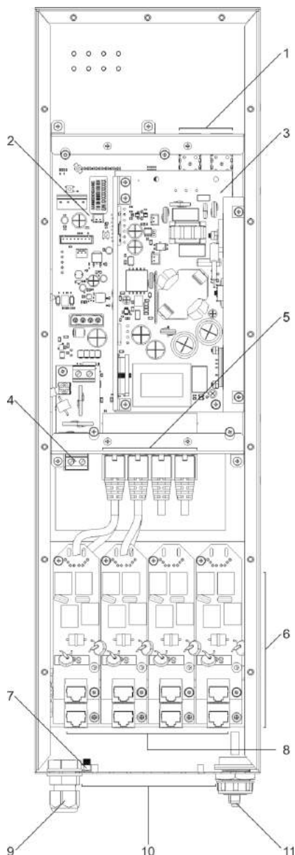
Рисунок 37 – Основные компоненты и разъемы MES3708P
