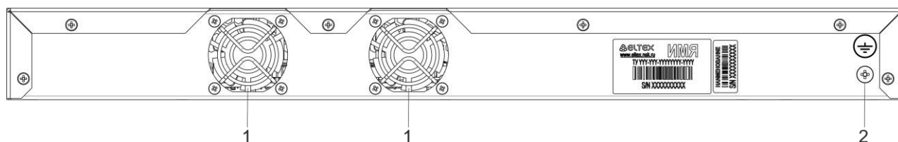
Рисунок 32 – Задняя панель MES2411X
