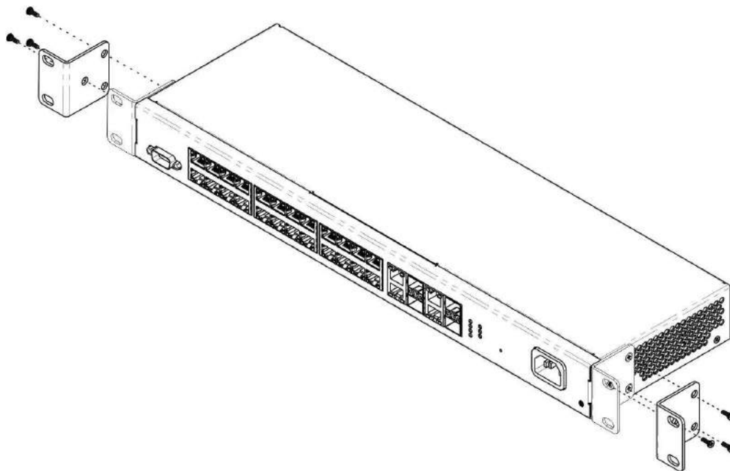
Рисунок 40 – Крепление кронштейнов
