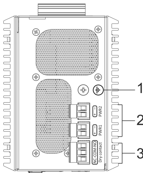
Рисунок 34 — Верхняя панель MES3710P
