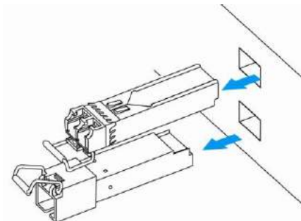
Рисунок 46 – Извлечение SFP-трансиверов
