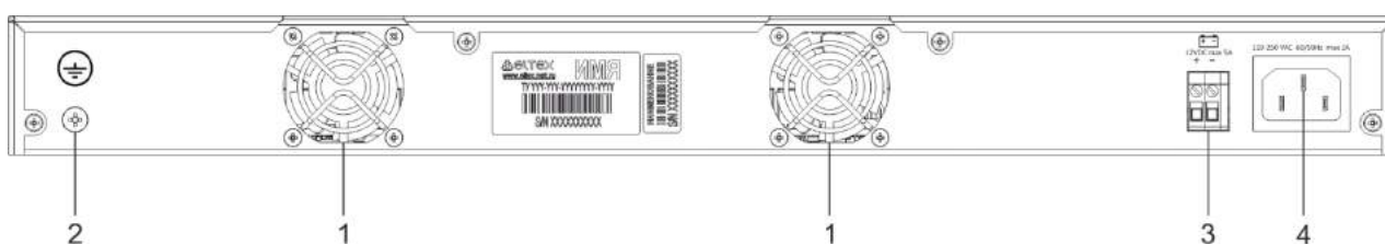
Рисунок 30 – Задняя панель MES2448B
