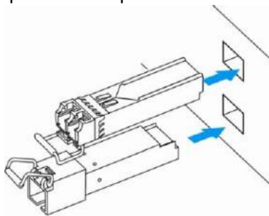
Рисунок 43 – Установка SFP-трансиверов
