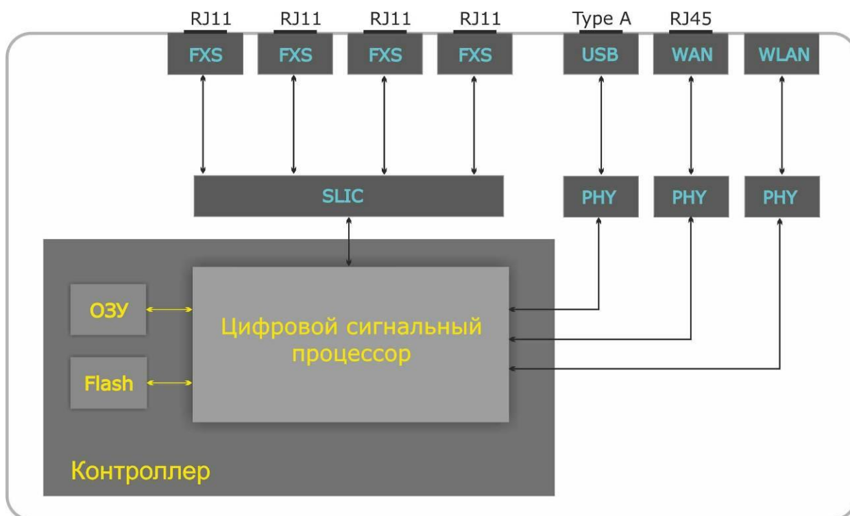
Рисунок 2 – Структурная схема TAU-4.IP
