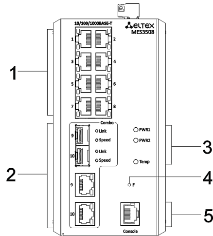
Рисунок 20 — Передняя панель MES3508
