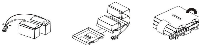
Рисунок 15 – Последовательность установки аккумуляторов в контейнер ИБП СГП2-010СБ Р102419
