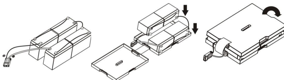
Рисунок 17 – Последовательность установки аккумуляторов в контейнер ИБП СГП2-020СБ Р104819
