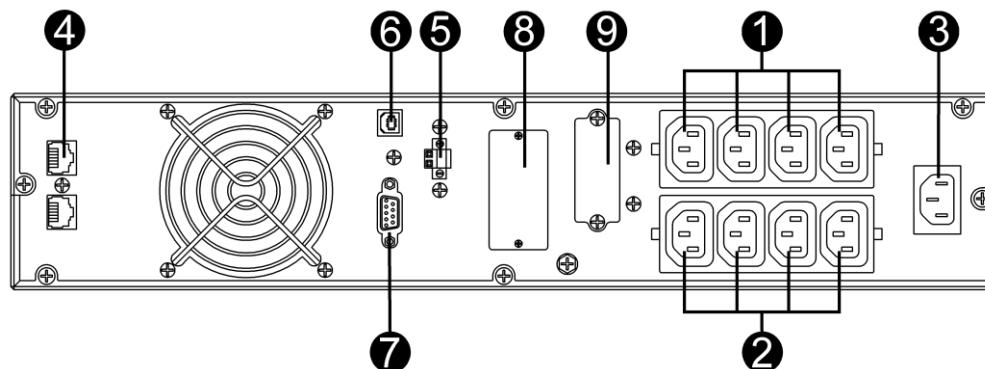
Рисунок 4 – Задняя панель СГП2-010СЕ / СГП2-010СБ, СГП2-015СЕ / СГП2-015СБ
