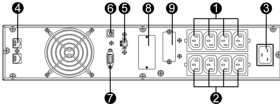
Рисунок 5 - Задняя панель ИБП СГП2-020СЕ / СГП2-020СБ
