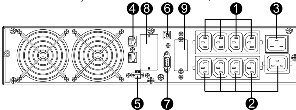
Рисунок 6 - Задняя панель ИБП СГП2-030СЕ / СГП2-030СБ
