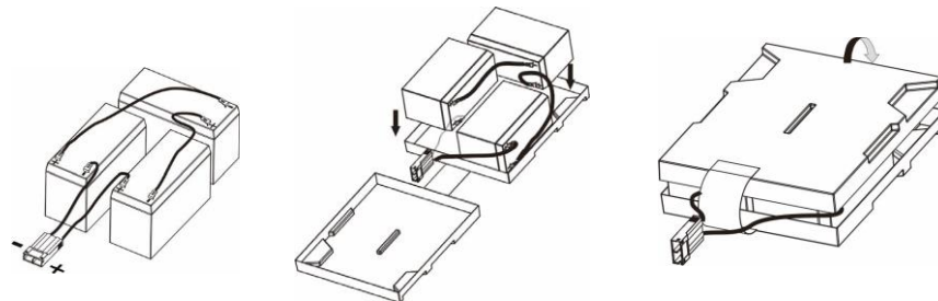
Рисунок 15 – Последовательность установки аккумуляторов в контейнер ИБП СГП2-010СБ Р102419
