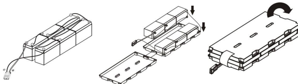
Рисунок 18 – Последовательность установки аккумуляторов в контейнер ИБП СГП2-020СБ Р107219 и СГП2-030СБ Р107219
