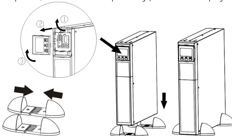
Рисунок 8 – Порядок установки ИБП в вертикальное напольное (настольное) положение
