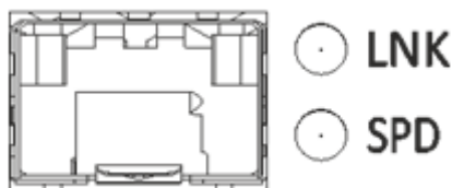
Рисунок 77 – Расположение индикаторов разъема SFP
