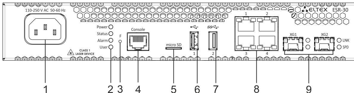
Рисунок 44 – Передняя панель ESR-30
