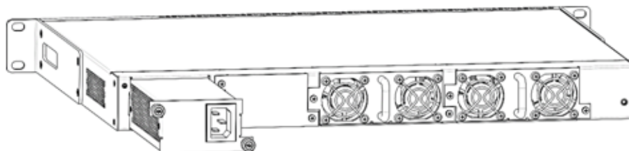
Рисунок 89 – Установка модулей питания
