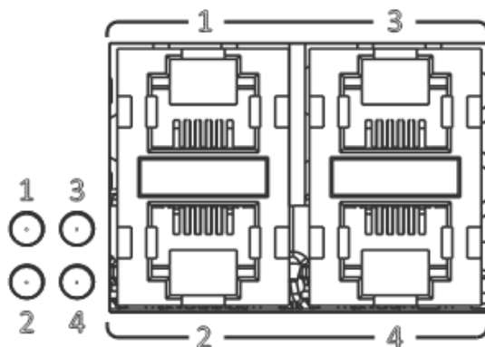
Рисунок 81 – Расположение индикаторов FXS-интерфейсов
