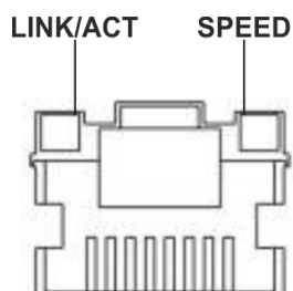
Рисунок 80 – Расположение индикаторов разъема RJ-45
