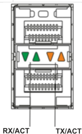
Рисунок 79 – Расположение индикаторов оптических интерфейсов
