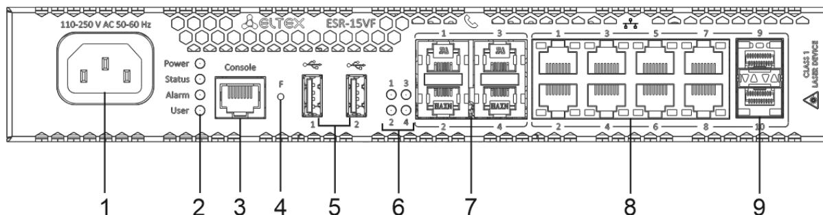
Рисунок 49 – Передняя панель ESR-15VF
