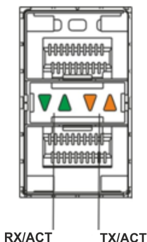
Рисунок 71 – Расположение индикаторов оптических интерфейсов
