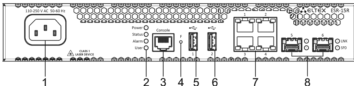
Рисунок 53 – Передняя панель ESR-15R
