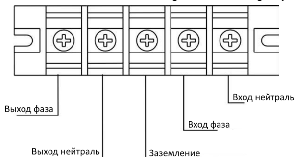
Рис.2 Подключение ИБП
