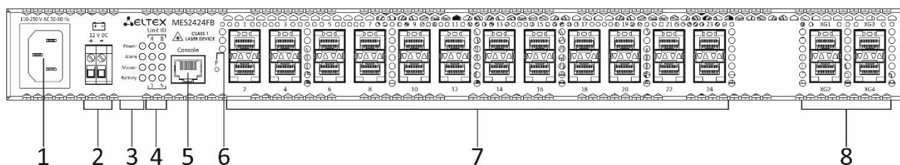
Рисунок 26 — Передняя панель MES2424FB
