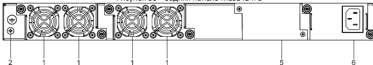
Рисунок 37 — Задняя панель MES3400-24, MES3400-48
