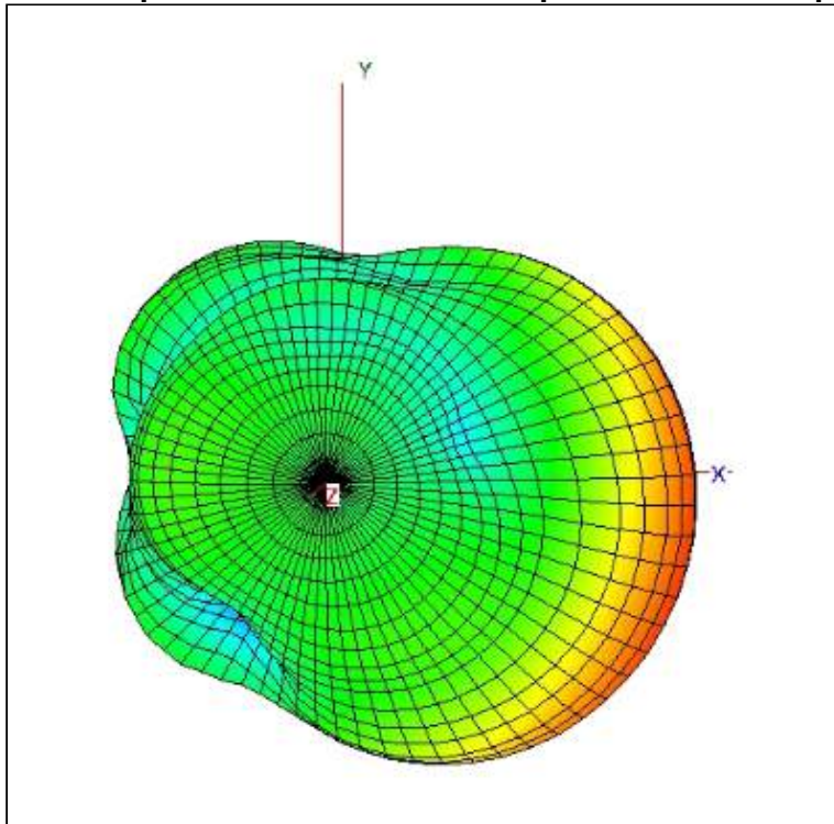
Диаграмма направленности антенны горизонтальной поляризации:
