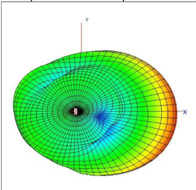
Диаграмма направленности антенны горизонтальной поляризации:
